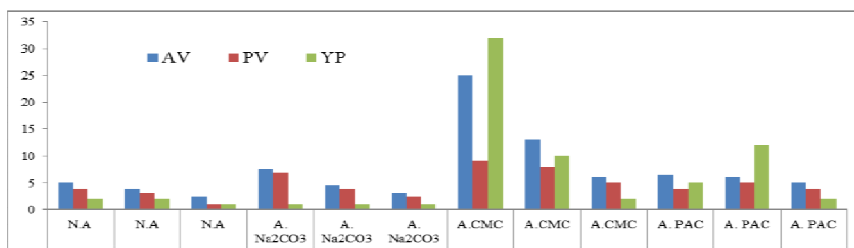
شکل ۱۱ ویژگی‌های سیال شناسی بنتونیت‌های ساده (N.A) و فعال شده (A) توسط \text{Na}_2\text{CO}_3 ، CMC و PAC.
