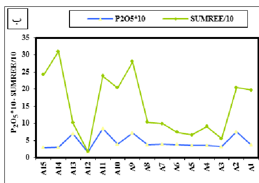
شکل ۶ الف) نمودار Eu/Eu^* - Ce/Ce^* - La/Y در تمام نمونه‌های پهنه‌های اسکارن باباعلی. ب) همبستگی بین عناصر خاکی نادر با P_2O_5 .
