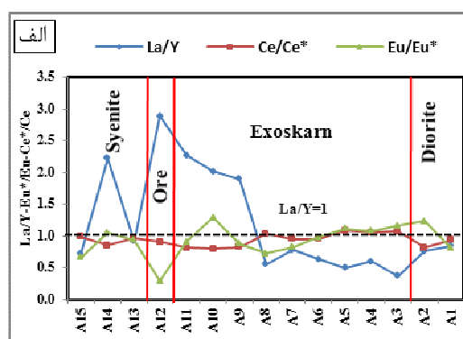
شکل ۶ الف) نمودار Eu/Eu^* - Ce/Ce^* - La/Y در تمام نمونه‌های پهنه‌های اسکارن باباعلی. ب) همبستگی بین عناصر خاکی نادر با P_2O_5 .
