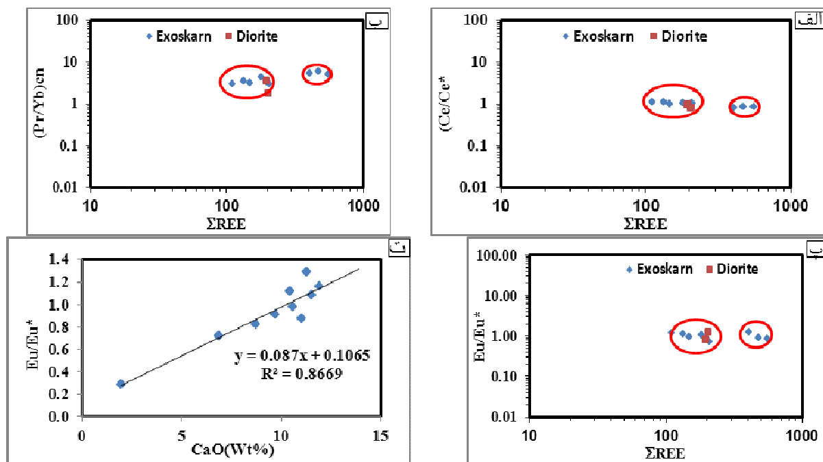
شکل ۷ الف تا پ: نمودارهای نشان دهنده نوع سیالات موثر در کانی‌سازی در اگرواسکارن در مقایسه با دیوریت میزبان که با توجه به پراکندگی نقاط به دو بخش می‌توان تقسیم کرد. (ت) همبستگی بین (Eu/Eu^*) - CaO در اگرواسکارن.
