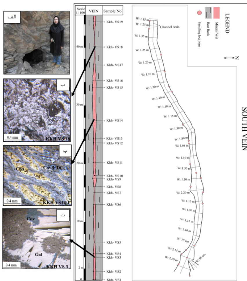
شکل ۵ نیمرخ طولی تونل حفر شده در رگه‌ی جنوبی (مختصات جغرافیای X: 51^{\circ} 26' 59'' ، Y: 36^{\circ} 12' 16'' ) و موقعیت نمونه‌های اخذ شده. الف: نما از دهانه‌ی ورودی تونل، ب: نمونه‌ی KKH-VS18 اکسیدهای آهن (هماتیت) در نور XPL. پ: نمونه‌ی 1/ KKH-VS14 رگچه کالکوپیریت در حال تبدیل به کوولیت در نور XPL. ت: نمونه‌ی KKH-VS3 گالن در حال تبدیل شدن به کوولیت و سروزیت (بافت جانشینی) در نور XPL.
