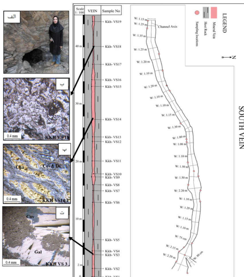
شکل ۵ نیمرخ طولی تونل حفر شده در رگه‌ی جنوبی (مختصات جغرافیای X: 51^{\circ} 26' 59'' ، Y: 36^{\circ} 12' 16'' ) و موقعیت نمونه‌های اخذ شده. الف: نما از دهانه‌ی ورودی تونل، ب: نمونه‌ی KKH-VS18 اکسیدهای آهن (هماتیت) در نور XPL. پ: نمونه‌ی 1/ KKH-VS14 رگچه کالکوپیریت در حال تبدیل به کوولیت در نور XPL. ت: نمونه‌ی KKH-VS3 گالن در حال تبدیل شدن به کوولیت و سروزیت (بافت جانشینی) در نور XPL.
