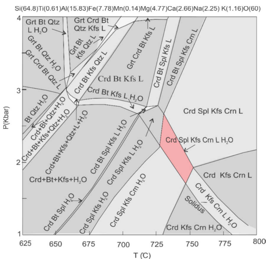
شکل ۱۳ شبه مقطع رسم شده برای میگماتیت‌های منطقه بروجرد با استفاده از برنامه Theriak/Domino نسخه ۲۰۱۲، منطقه صورتی مجموعه کانی‌های میگماتیت‌های بروجرد در شرایط اوج دگرگونی را نشان می‌دهد.
