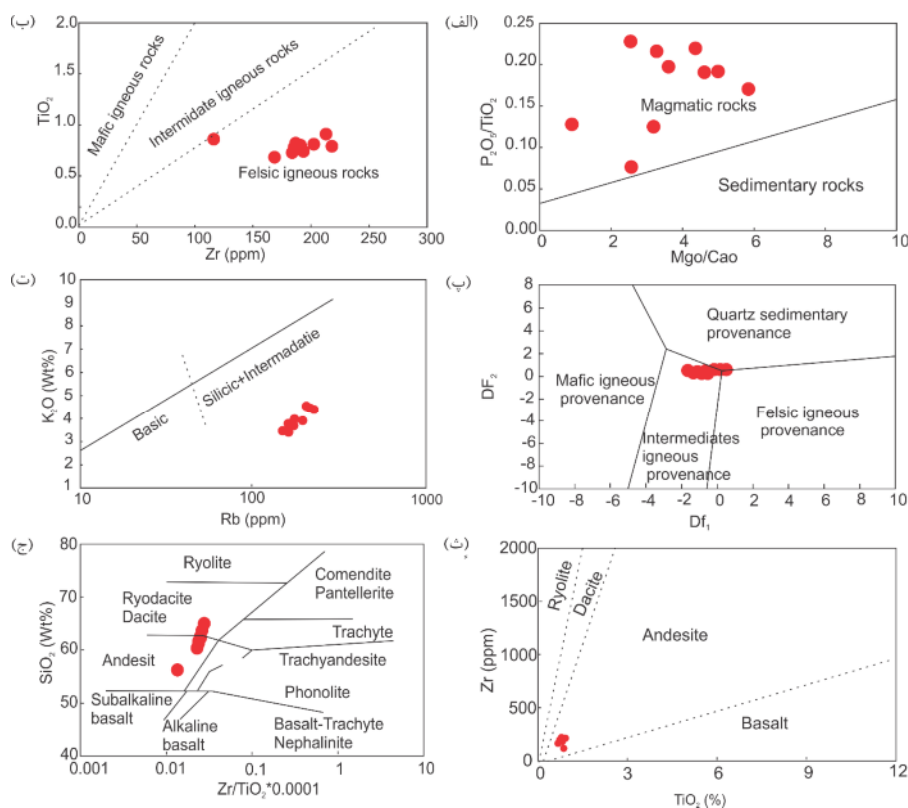
شکل ۴ الف) نمودار تفکیک سنگ خاستگاه آذرین و رسوبی [۱۴] ب) نمودار \text{TiO}_2 نسبت به Zr [۱۵] که نشان می‌دهد که میگماتیت‌های منطقه بروجرد خاستگاه آذرین فلسی داشته‌اند. پ و ت) نمودارهای ارائه شده در مرجع [۱۶] که بیانگر خاستگاه حدواسط تا اسیدی برای رسوبات اولیه میگماتیت‌های منطقه بروجرد است. ث) نمودار \text{Zr}-\text{TiO}_2 [۱۷] و ج) نمودار دو متغیره \text{SiO}_2 نسبت به \text{Zr}/\text{TiO}_2 \cdot 0.0001 [۱۸] که نشان می‌دهند که سنگ خاستگاه میگماتیت‌های بروجرد براساس شیمی عناصر غیر متحرک سنگ‌های آذرین حدواسط مانند آندزیت تا داسیت و ریوداسیت است.
