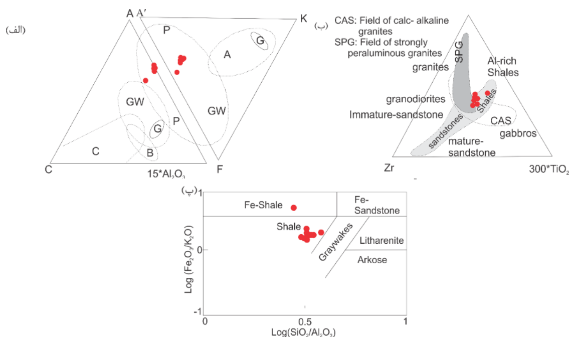
شکل ۳ الف) نمودار A'FK-ACF [۱۲] برای تعیین سنگ مادر میگماتیت‌های بروجرد. P: سنگ‌های پلیتی، GW: ماسه سنگ تیره G: گرانیت، C: سنگ‌های آهکی، B: بازالت، A: آندزیت. ب) نمودار سه تایی \text{Zr}-15 \cdot \text{Al}_2\text{O}_3-\text{TiO}_2 \cdot 300 [۲۴] که بر اساس آن سنگ مادر میگماتیت‌ها از نوع شیل است. پ) رده بندی مرجع [۱۳] که بر اساس آن سنگ مادر میگماتیت‌ها از نوع شیل است.
