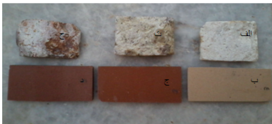
شکل ۴ نمونه KA1. الف: قبل از آزمون پخت، ب: بعد از آزمون پخت؛ آزمایشی و نمونه KA2. ت: قبل از پخت، ازمایشی ج: بعد از پخت؛ آزمایشی و نمونه BK300. ح: قبل از آزمون پخت، د: بعد از آزمون پخت.
