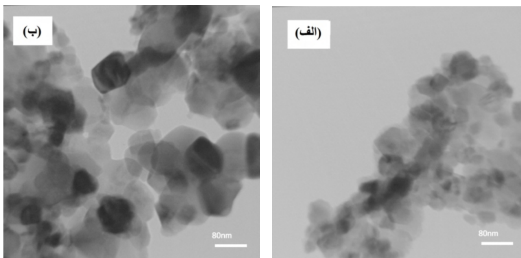
شکل ۳ تصاویر TEM نمونه‌های (الف) خالص و (ب) با ۴/۱ ناخالصی آلومینیوم.
