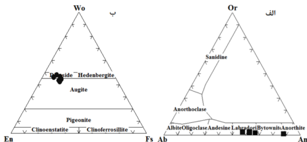
شکل ۴ الف) جایگاه ترکیبی پلاژیوکلازهای موجود در گدازه‌های بازیک مورد بررسی بر نمودار تقسیم‌بندی فلدسپارها [۳۰] و ب) نمودار سه‌تایی \text{En-Wo-Fs} [۳۵] برای رده‌بندی کلینوپیروکسن‌ها.
