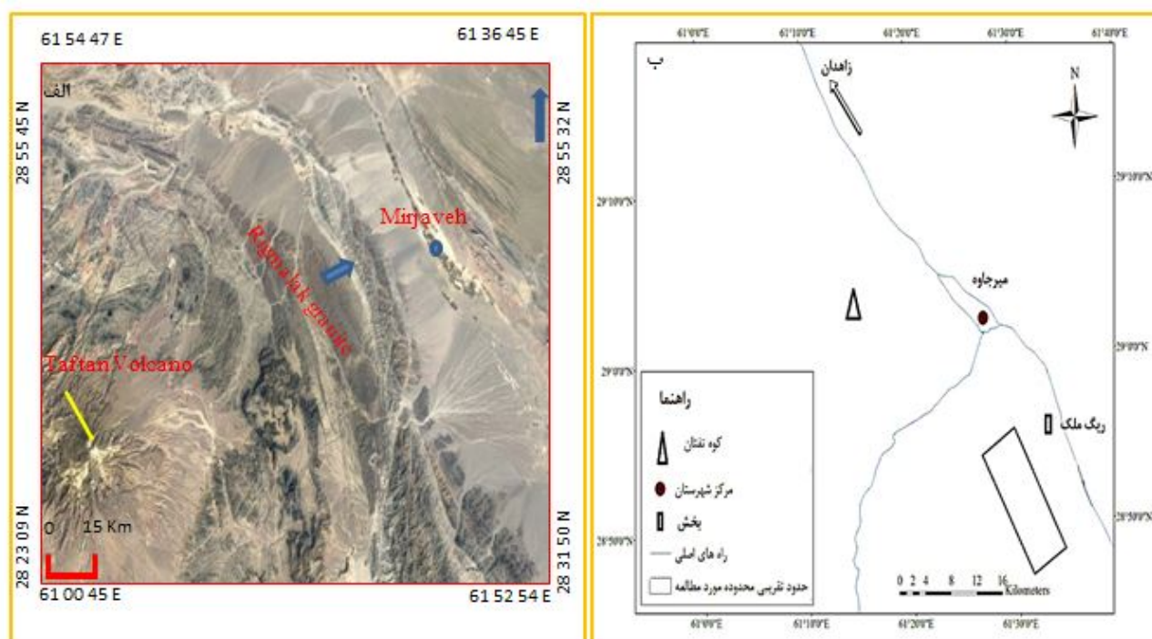
شکل ۱ الف: جایگاه گرانیتهوئید ریگ ملک واقع در شرق و شمال شرق آتشفشان تفتان، جنوب شرق ایران (بر تصاویر ماهواره ای (ETM+، ب- راه های دسترسی به منطقه.
