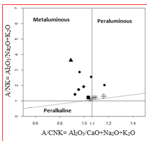
شکل ۹ جایگاه نمونه‌های سنگی منطقه ریگ ملک بر نمودار شاخص آلومینیوم [۱۱، ۳۴] که بیشتر نمونه‌ها در گستره متآلومین و کمی پرالومین قرار دارند.
