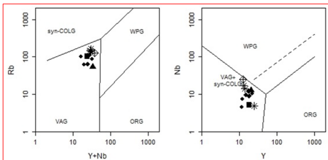
شکل ۱۱ نمودارهای \text{Nb}/\text{Y} و \text{Rb}/\text{Y+Nb} [۳۸] که براساس آنها، سنگ‌های مورد بررسی در گستره گرانیت‌های قوس‌های آتشفشانی قرار دارند.
