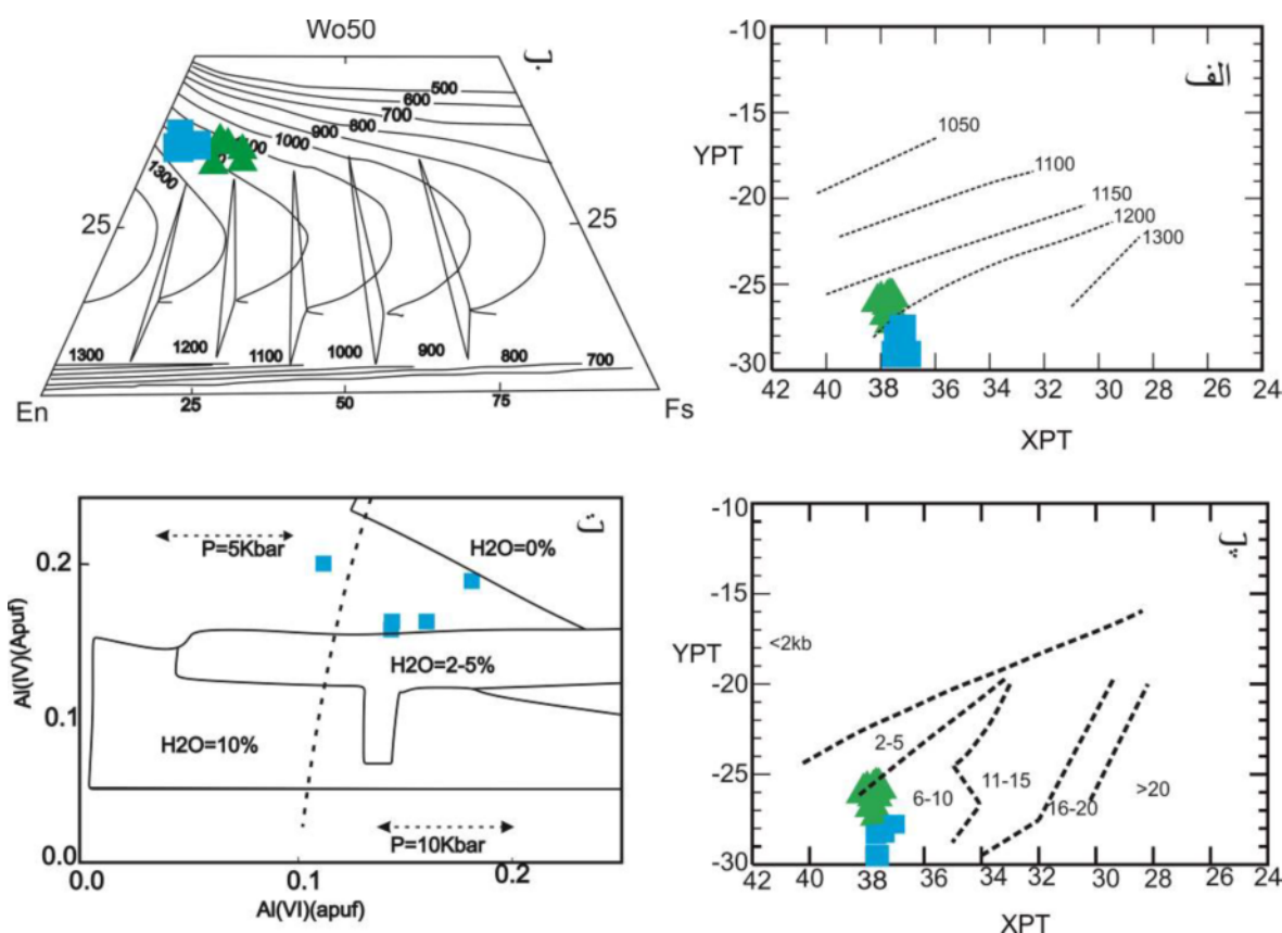
شکل ۷ تعیین دمای پیروکسن‌های منطقه جویبار با استفاده از روش مرجع [۳۳] و (ب) نمودار Wo-En-Fs [۳۴]. (پ) تعیین فشار تبلور پیروکسن با استفاده از روش مرجع [۳۳] و (ت) بررسی فشار و مقدار آب موجود در ماگما بر پایه شیمی کانی پیروکسن [۳۸]. علائم مشابه شکل ۵ است.
