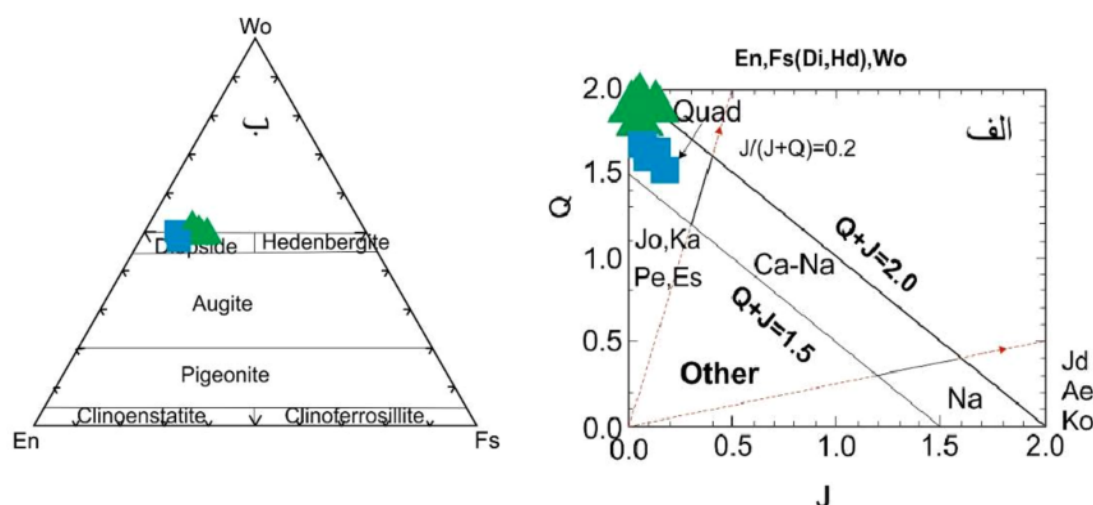
شکل ۵ رده‌بندی پیروکسن‌های منطقه جویار: الف) ترکیب کلینوپیروکسن‌ها در نمودار Q نسبت به J [۱۸] و ب) نمودار En-Fs- WO [۱۹]. (نمونه‌های دایک دیابازی: نشان‌دهنده نمونه‌های دایک لامپروفیری)
