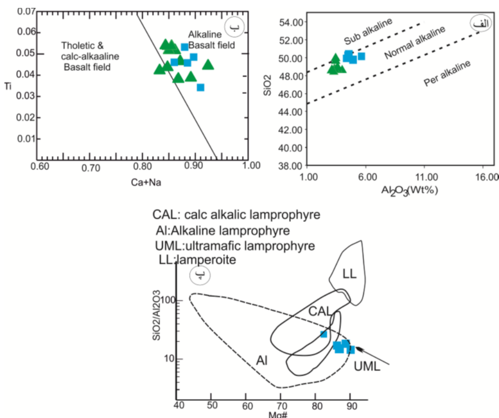
شکل ۶ تعیین سری ماگمایی و جایگاه زمین‌ساختی نمونه‌ها با استفاده از ترکیب شیمیایی پیروکسن در (الف) نمودار SiO 2 به نسبت به Al 2 O 3 [۲۰]، (ب) نمودار Ca+Na در مقابل Ti [۵] و (پ) نمودار شناسایی سری ماگمایی لامپروفیرها [۲۴].
