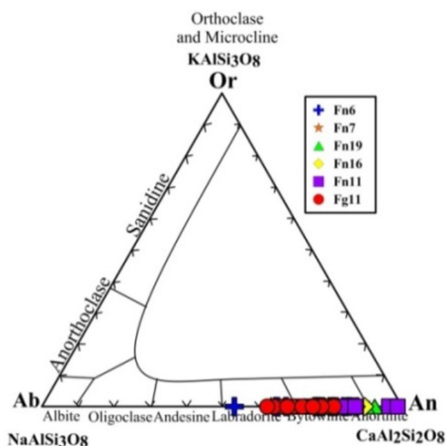
شکل ۸ جایگاه پلاژ و کلازهای سنگ‌های دیو، تپه کر تاسه بسین جنوب غرب سبزوار در نمودار سه تایی، رده‌بندی فلدسپارها [۳۳].
