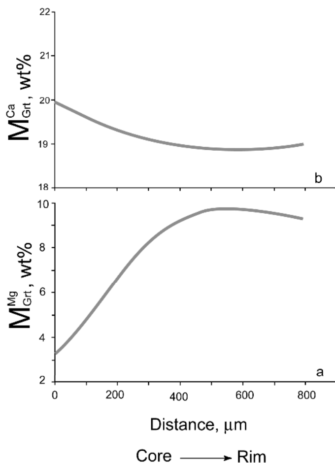
شکل ۴ منطقه‌بندی شیمیایی کلسیم و منیزیم برای گارنت در سنگ‌های رسی دگرگون شده منطقه‌ی جندق (برگرفته از [۱۶]).
