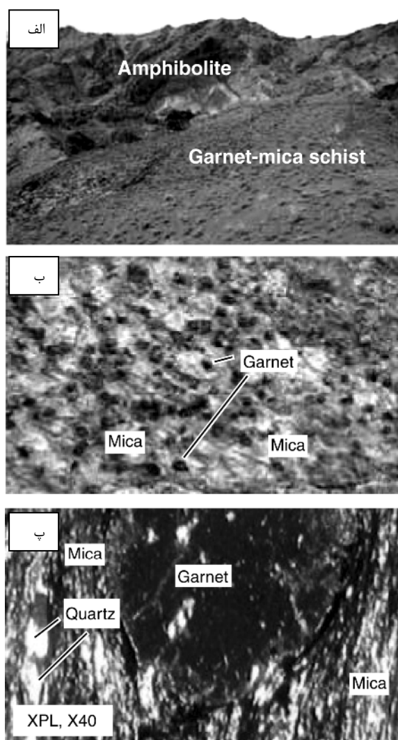
شکل ۲ سنگ‌های دگرگون منطقه‌ی جندق. الف. برونزد گارنت- میکا شسیت و آمفیبولیت. ب. گارنت‌های نسبتاً درشت در گارنت- میکا شسیت. پ. مقطع میکروسکوپی از گارنت- میکا شسیت. برگوازی سنگ از بالا به پائین مشخص است. تصاویر برگرفته از [۱۶] با تغییرات.
