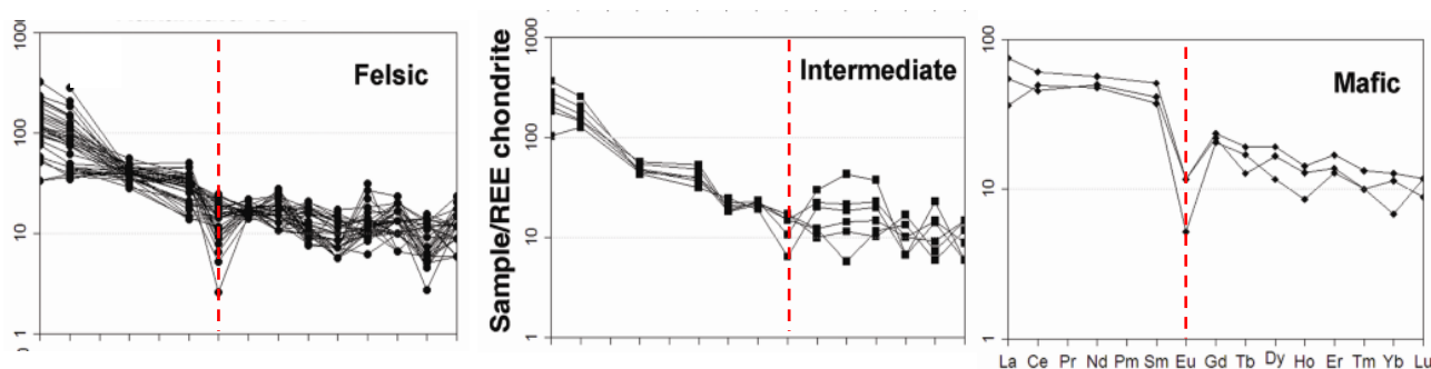
شکل ۱۲ الگوی بهنجار شده عناصر خاکی نادر سنگ‌های گرانودیوریتی-مونزوگرانیته، دیوریتی و گابرویی منطقه مورد بررسی [۶۳].
