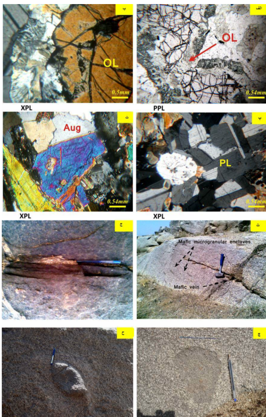
شکل ۳ الف، ب، پ- تصاویری از مقاطع نازک تهیه شده از توده گابرو-دیورتی بخش شمالی کوه تنگساران که به ترتیب بیانگر لبه واکنشی الیوین با کانی‌های در بر گیرنده و رسوب کانی‌های کدر در درز و ترک‌های سطح آن در اثر برداشته شدن فشار از روی مجموعه (مذاب) دورگه حمل کننده ی آن طی صعود (الف، ب) و حضور پلاژیوکلازها در کنار آنها در مجموعه‌ای با بافت دلریتی و متراکم است، ت- تصویری از دیورت‌های پیروکسن دار روستای قلعه مهدی خان و ماکل دوتایی مشخص در کانی اوژیت، ث- تصویری از رگه بازیک سرشار از کانی هورنبلند سبز و بیوتیت که در کنار برونومهای میکروانه ای عدسی شکلی که راستای محور طولی موازی با راستای برگوارگی سنگ میزبان دارند قرار گرفته است، ج- بیگانه بلورهایی از خاستگاه واحدهای شیستی کنار توده گرانودیوریتی که در برابر گرمای ماگمای میزبان مقاومت نموده و کاملاً هضم نشده‌اند و چنان که دیده می‌شود، حتی لایه بندی شیست خاستگاه همچنان پابرجاست، چ- برونوم ماگمایی اسیدی یا میکروگرانیتوئیدی و ح- برونوم ماگمایی بازیک دوکی شکل (OL: الیوین، Aug: اوژیت و PL: پلاژیوکلاز).
