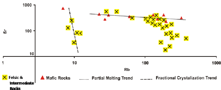
شکل ۱۱: نمودار لگاریتمی عنصر سازگار در برابر ناسازگار [۶۱]. برای سنگ‌های اسیدی و بازیک منطقه، دو نوع روند برای نمونه‌های اسیدی و بازیک این منطقه دیده می‌شود: ۱- روند نزدیک به قائم و روند منحنی شکل نزدیک به قائم برای نمونه‌های اسیدی و حدواسط منطقه که بیانگر تبلور تدریجی همراه با مقداری آرایش ماگمایی است و ۲- روند نزدیک به افق که بیانگر ذوب بخشی سنگ‌های بازیک است.
