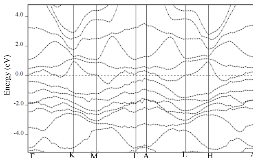
شکل ۷ ساختار نواری ZnO:Al انرژی فرمی در مبدا با خط چین مشخص شده است. انتقال انرژی فرمی به داخل نوار رسانش مشهود است.
