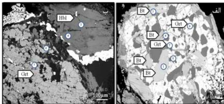
شکل ۶ نقاط تجزیه شده توسط ریزکاوالکترونی نشان دهنده الف) وجود بیوتیت در گارنت‌های متاپلیت‌ها و ب) همجواری هورنبلند و گارنت در گارنت آمفیبولیت‌های منطقه گل‌گهر.
