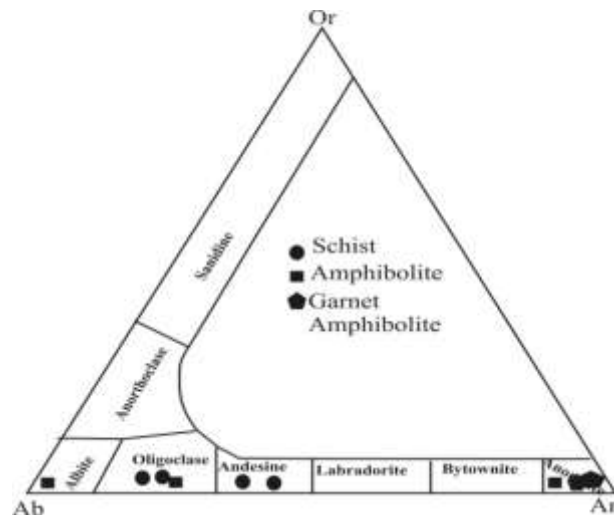
شکل ۴ رده‌بندی فلدسپارها در سنگ‌های دگرگونی منطقه گل‌گهر بر اساس نمودار مرجع [۱۶].
