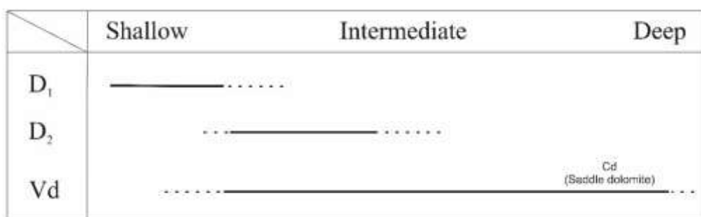
شکل ۷ توالی همزادی دولومیت‌های سازند سبزار در برش خرو.
