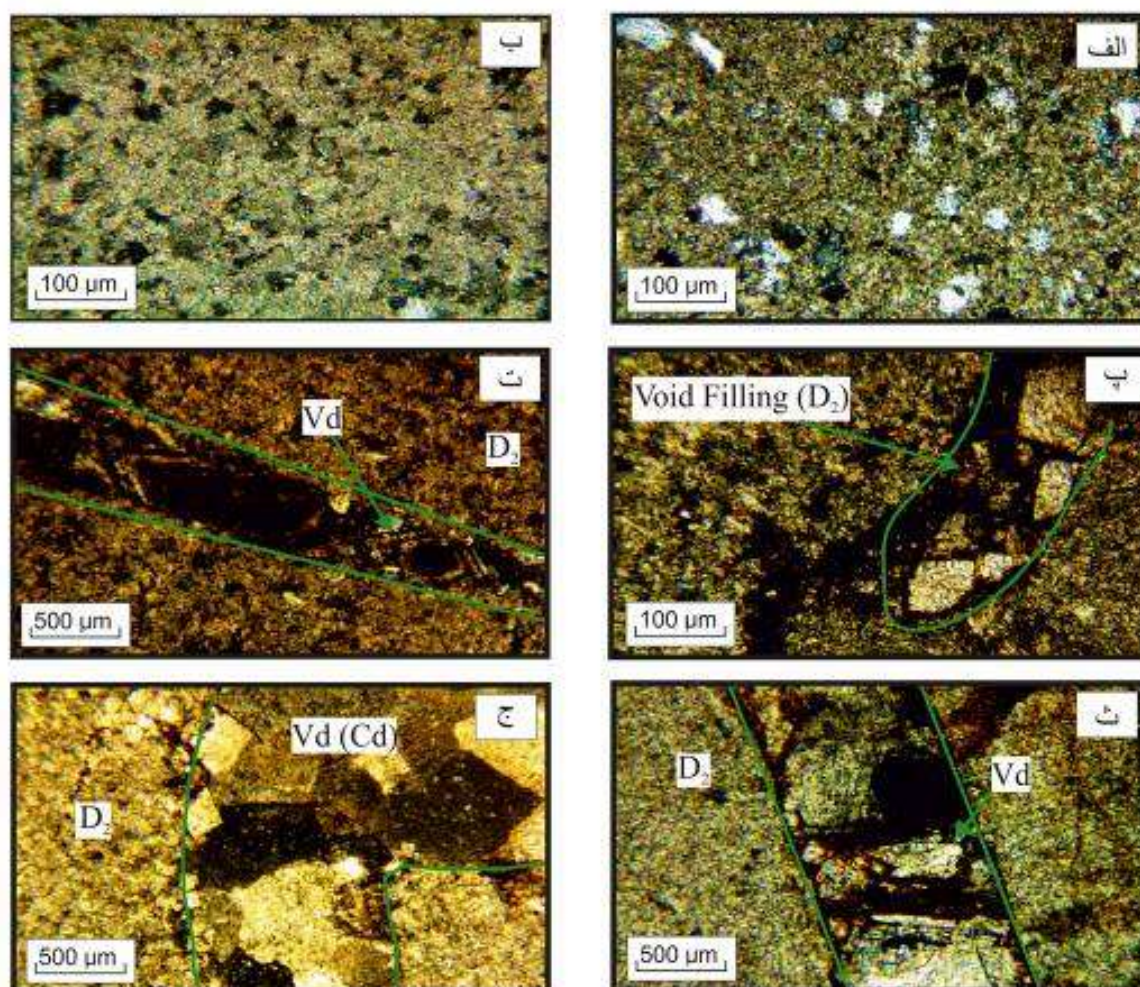
شکل ۵ تصاویر مقاطع میکروسکوپی دولومیت‌های سازند سبزار: (الف) دولومیت نوع D_1 دارای بافت غیر مسطح-a (موزایک نامنظم) همراه با ذرات کوارتز، (ب) دولومیت نوع D_2 دارای بافت غیر مسطح-a (موزایک نامنظم)، (پ) دولومیت نوع D_2 بصورت حفره پرکن دارای بافت مسطح-e (موزایک منظم)، (ت) دولومیت رگه‌ای Vd دارای بافت مسطح-e (موزایک منظم) که توسط اکسید آهن قسمتی از رگه پوشیده شده است و دولومیت نوع D_2 دارای بافت غیر مسطح-a (موزایک نامنظم) (ث) دولومیت رگه‌ای Vd دارای بافت مسطح-e (موزایک منظم) و مسطح-s (موزایک نیمه منظم) و دولومیت نوع D_2 دارای بافت غیر مسطح-a (موزایک نامنظم) و (ج) دولومیت رگه‌ای Vd دارای بافت دولومیت زین اسبی شکل، (Cd: Saddle dolomite) و دولومیت نوع D_2 دارای بافت غیر مسطح-a (موزایک نامنظم).
