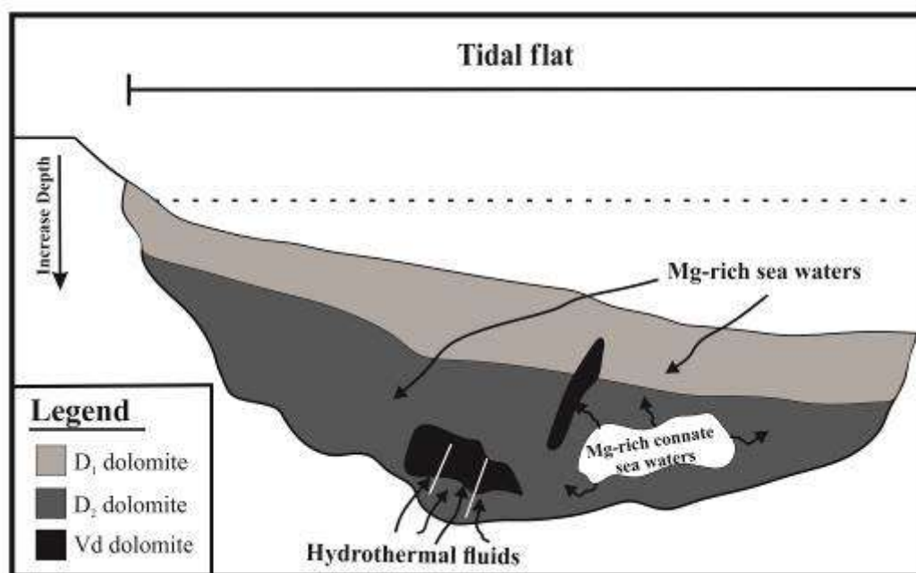
شکل ۸ مدل دولومیتی‌شدن سازند سبزار در برش خرو.
