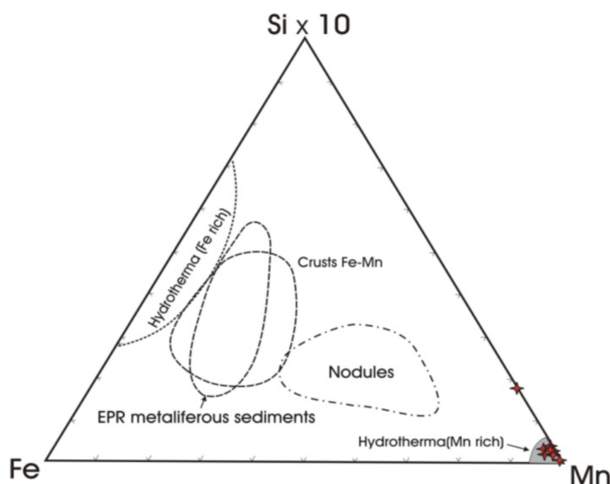
شکل ۱۰ ترکیب شیمیایی پیرولوئیت در نمودار سه قطبی 10 \text{ Mn} - \text{Fe} - \text{Si} \times 10
