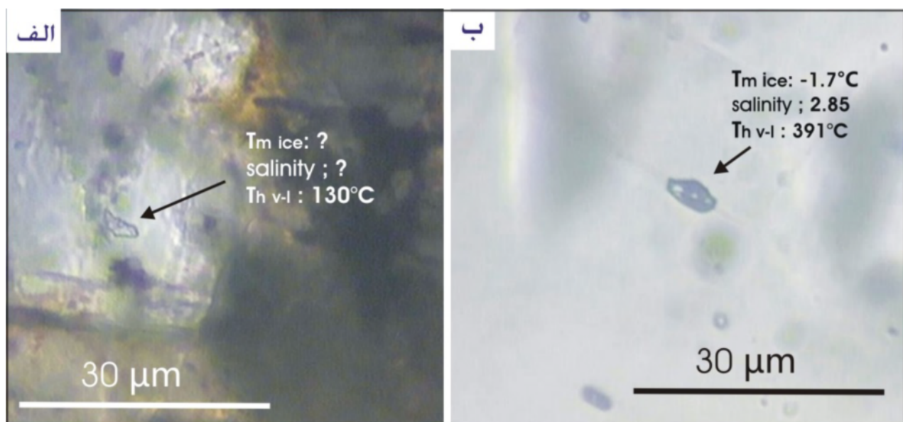
شکل ۹ تصاویر میکروسکوپی از میانبرهای سیال دوفازی مورد بررسی. الف: میانبرهای سیال دوفازی بخار و مایع در اسپسارتیت و ب: میانبرهای سیال دوفازی بخار و مایع در کوارتز. بنظر میرسد که میانبرهای اسپسارتیت ثانوی باشند، زیرا در شکستگی بلور به دام افتاده‌اند.
