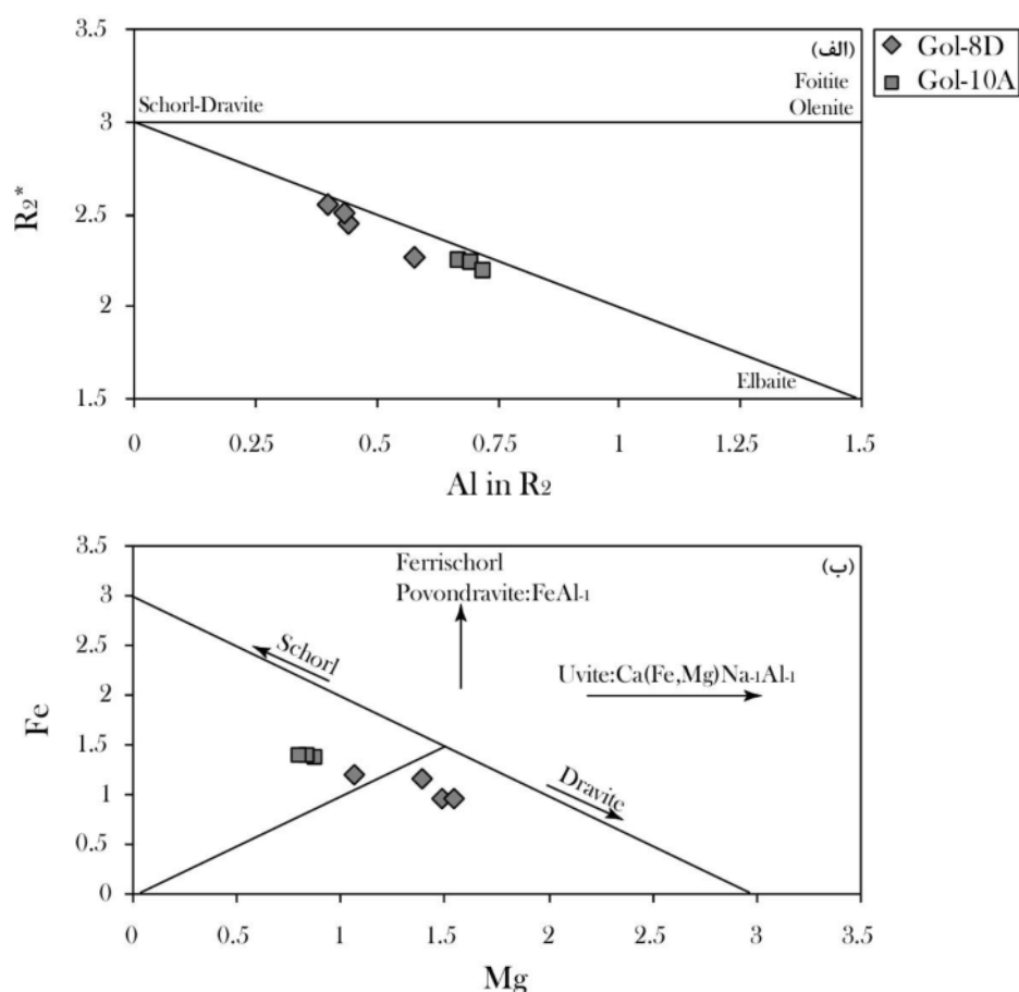
شکل ۷ الف) نمودار R_2^* نسبت به Al در R2 و R_2^*=Fe+Mg+Mn در Al ( R_2=Al+1.33Ti+Si-12 ) و (ب) نمودار Fe نسبت به Mg برای تورمالین‌های مورد بررسی (برگرفته از مرجع [۳۸]). هر دو نمودار جانشینی Al در جایگاه Y برای تورمالین‌های منطقه گلپایگان را نشان می‌دهد.
