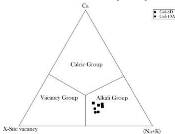
شکل ۳ رده‌بندی تورمالین‌ها بر اساس نمودار \text{Ca-(Na+K)} تهیجای جایگاه \text{X} (برگرفته از مرجع [۹]).
