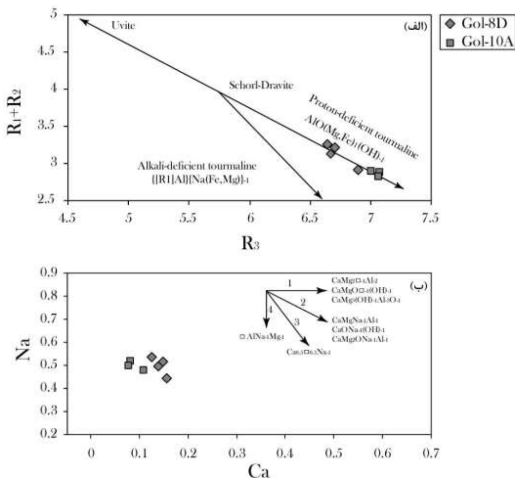
شکل ۶ الف) جانشینی کاتیون‌ها در تورمالین‌های مورد بررسی با استفاده از نمودارهای R_1+R_2 نسبت به R_3 ( R_2=Fe+Mg+Mn , R_1=Ca+Na ) و (ب) بررسی جانشینی کاتیون با استفاده از نمودار Na نسبت به Ca (برگرفته از مرجع [۳۷]).
