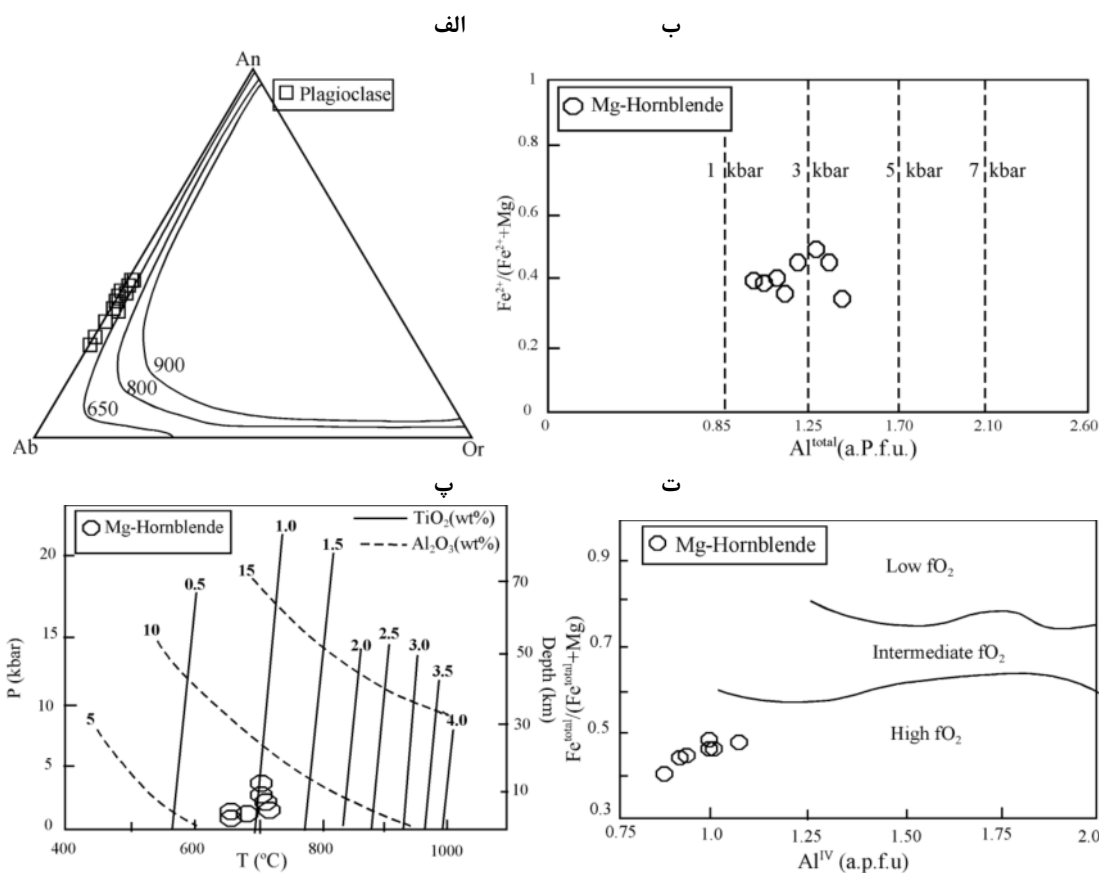
شکل ۵ الف- نمودار آنورتیت-آلیت-ارتوکلاز به منظور دماسنجی کانی‌های فلدسپار موجود در توده گرانیتی اسماعیل آباد در فشار ۱ کیلو بار [۱۶]. ب- نمودار فشارسنجی آمفیبول‌های موجود در این گرانیت‌ها [۱۷]. پ- نمودار تغییرات دما-فشار-عمق بر اساس مقدار \text{TiO}_2 و \text{Al}_2\text{O}_3 موجود در آمفیبول‌ها [۱۸]. ت- بررسی گریزندگی اکسیژن ماگمای مولد گرانیت‌های مورد بررسی براساس ترکیب آمفیبول‌ها [۱۹].
