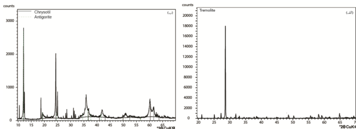
شکل ۴ قله‌های شناسایی شده بر اساس مقادیر d و \theta وابسته به (الف) ترمولیت در سنگ دارای آزبست آمفیبول، (ب) کریزوتیل و آنتی‌گوریت در سرپانتینیت‌های تخت سلیمان.
