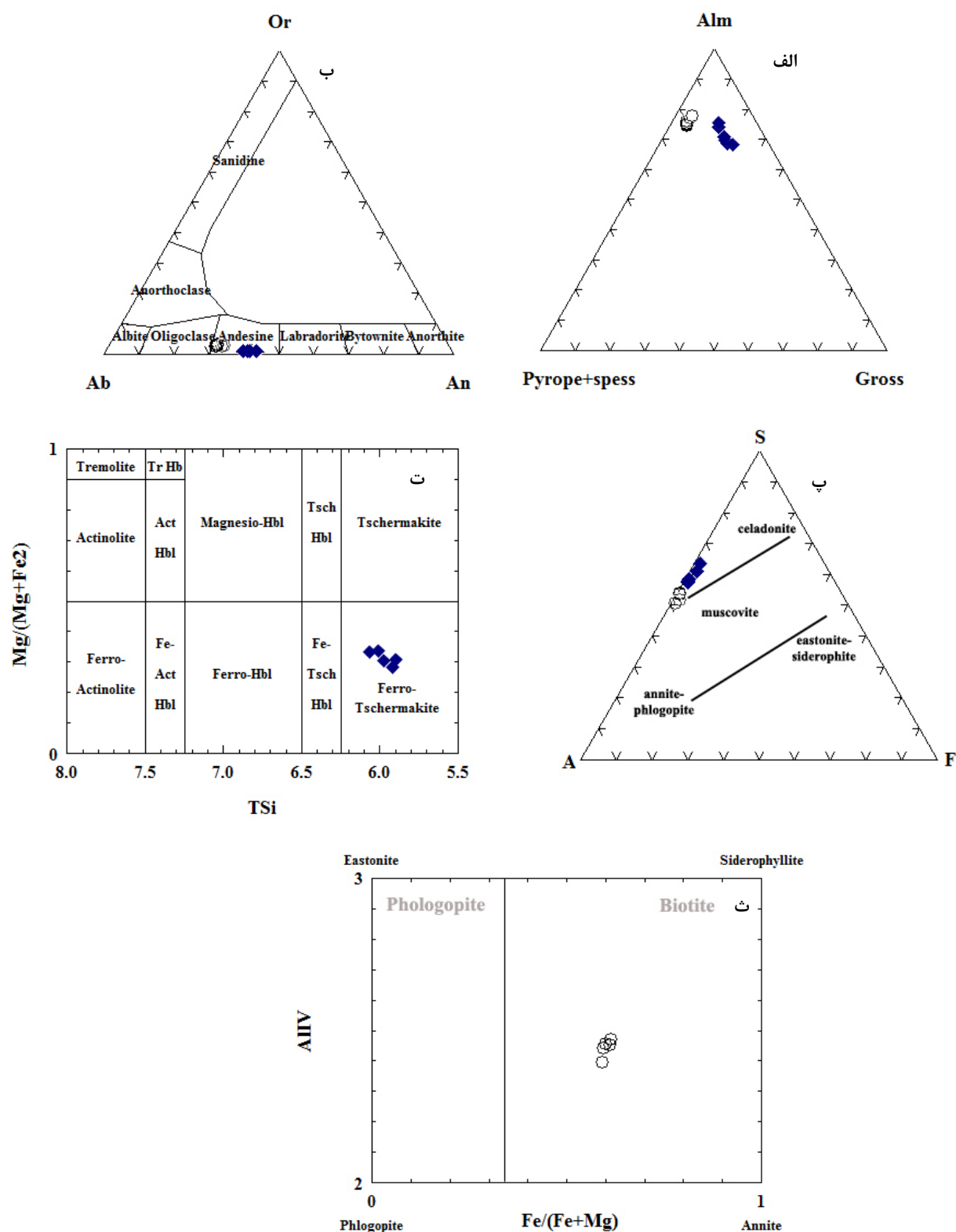
شکل ۷ (الف) جایگاه بلورهای گارنت در نمودار آلماندن - گروسولار - پیروپ + اسپسارتن [۱۲]، (ب) جایگاه کانی‌های پلاژیوکلاز در نمودار آنورتیت - آلبیت - اورتوز [۱۳]، (پ) جایگاه ترکیب شیمیایی بلورهای میکای سفید در نمودار سه تایی \text{SiO}_2\text{-Al}_2\text{O}_3\text{-FeO} [۱۴]، (ت) جایگاه بلورهای آمفیبول در نمودار مرجع [۱۵] و (ث) ترکیب شیمیایی بلورهای بیوتیت در نمودار مرجع [۱۳].
