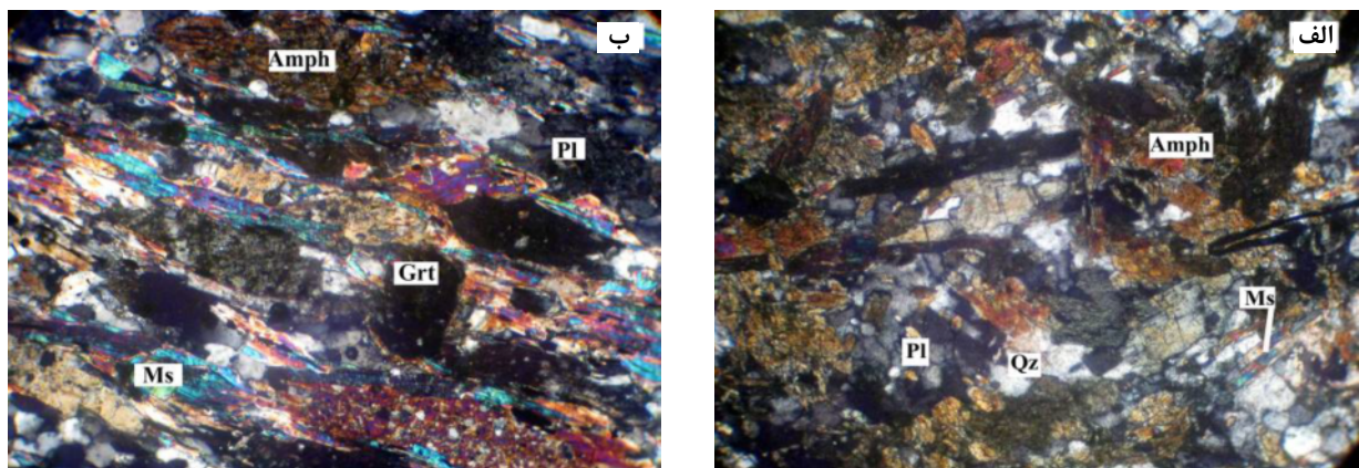
شکل ۵ تصاویر میکروسکوپی از سنگ‌های متنازیتی مورد بررسی (در نور XPL).
