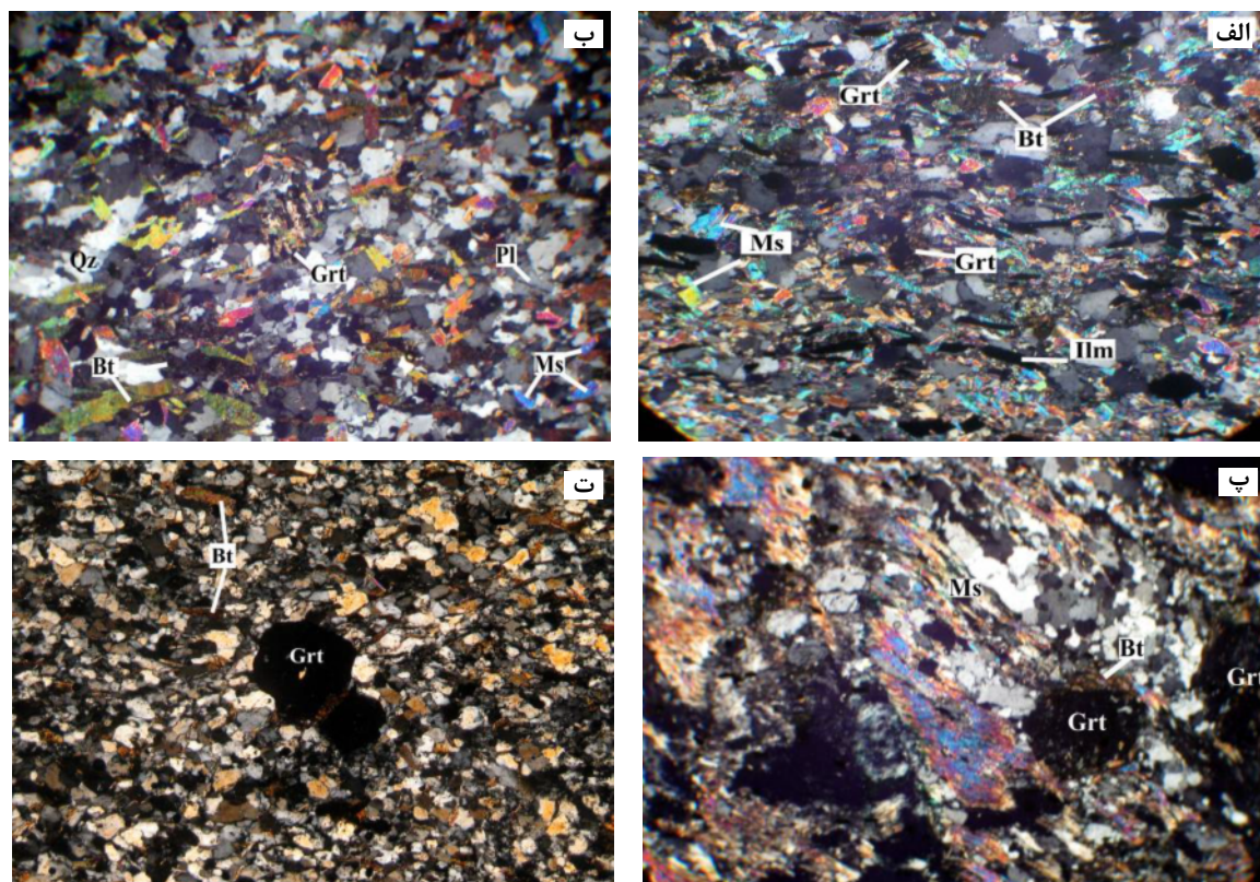
شکل ۶ تصاویر میکروسکوپی از سنگ‌های متنازیتی مورد بررسی (در نور XPL).
