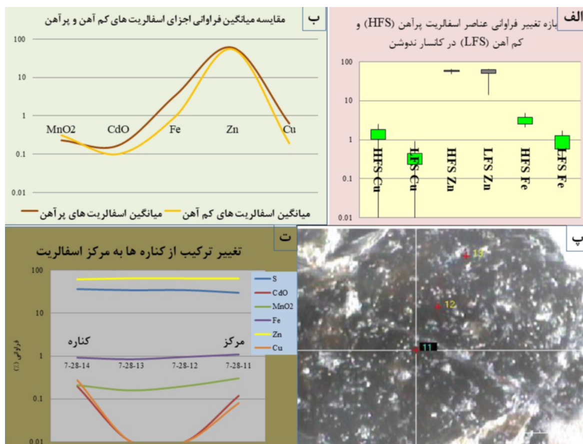
شکل ۶ الف) گستره تغییرات برخی عناصر در اسفالریت کم آهن (LFS) و پرآهن (HFS)، ب). مقایسه میانگین برخی عناصر در اسفالریت‌های کم آهن و پرآهن، پ) تصویر نقاط تجزیه شده بر یک اسفالریت کم آهن و ت) نمایش تغییرات عناصر آن.
