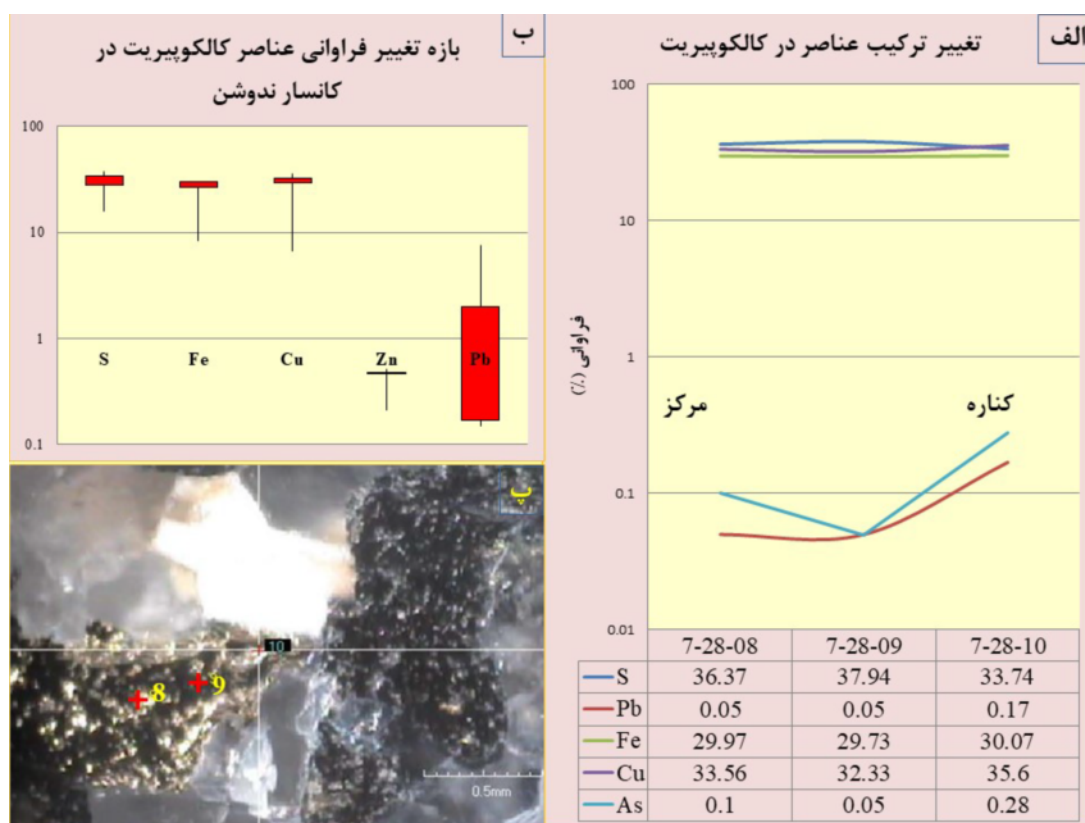
شکل ۷ الف) تغییرات مرکز به کناره در کالکوپیریت، ب) گستره فرآوانی عناصر موجود در یکی از نمونه های کالکوپیریت و پ) جایگاه برخی نقاط تجزیه شده بر آن.
