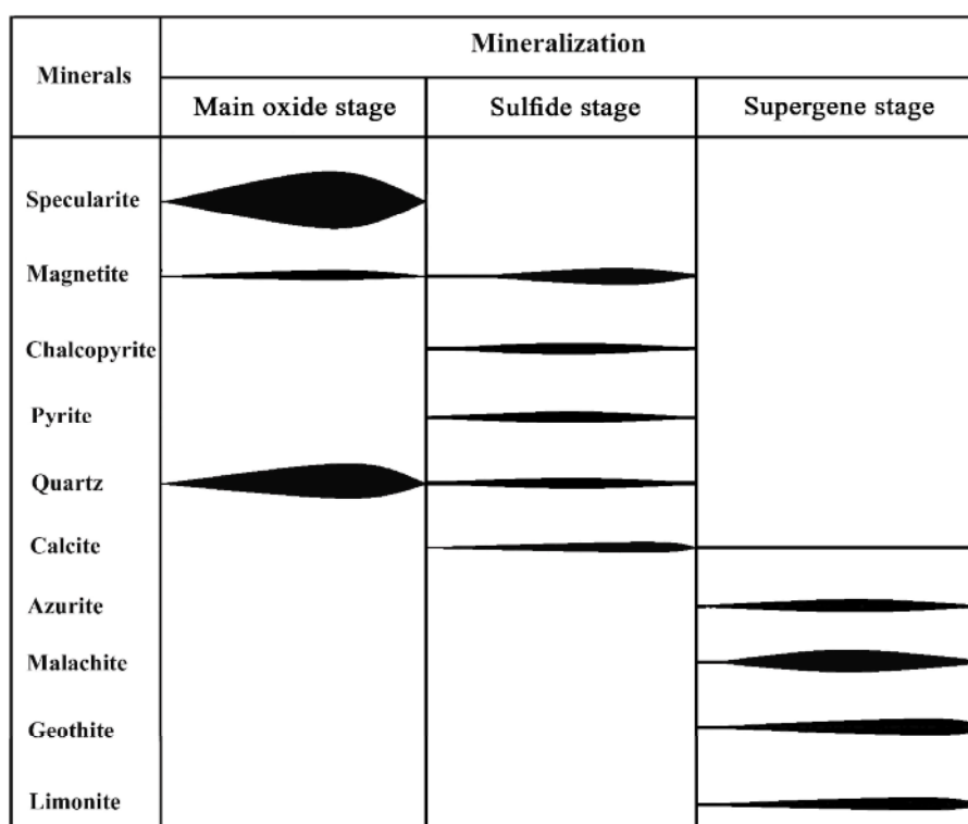
شکل ۲۰ دنباله‌ی تشکیل دوگانه‌ی کانسار آهن رشتخوار.
