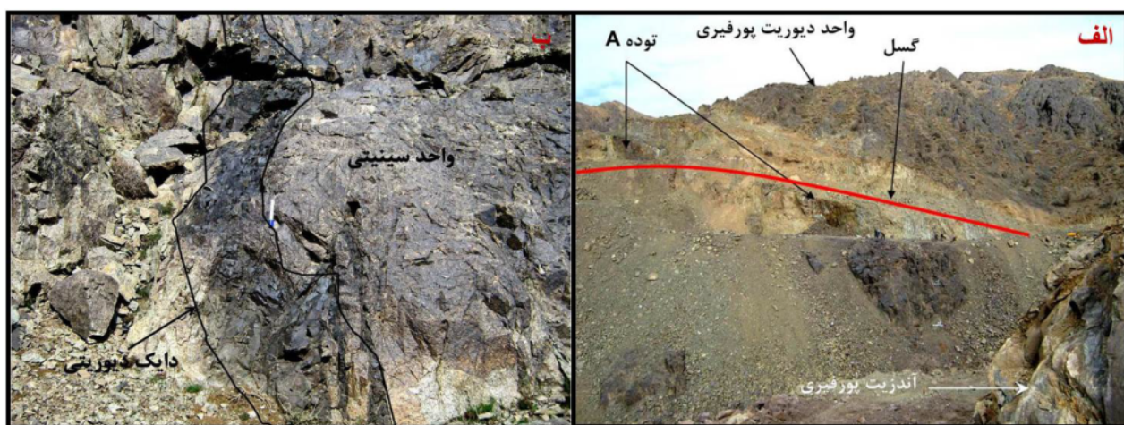
شکل ۶ الف) نمایی از توده‌ی معدنی A و واحد دیوریت پورفیری، ب) دایک‌های دیوریتی در واحدهای سینی با راستای N15W.
