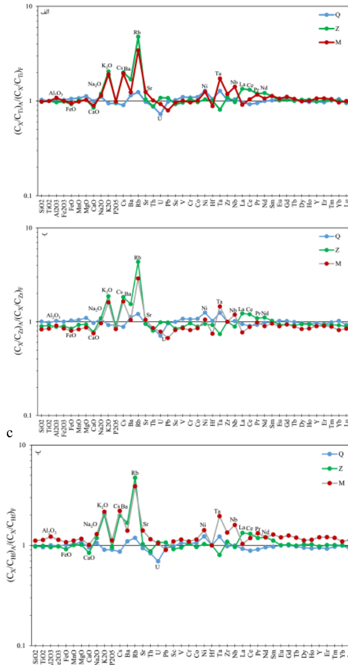
شکل ۷ نمودارهای مدل سازی و بهنجارش عناصر اصلی و جزئی نسبت به عناصر بایستار (الف) Ti، (ب) Zr، و (پ) Hf. علایم Q، Z، M به ترتیب علامت اختصاری مربوط به نمونه‌های سه کوه قلعه‌برد، پیازه و کوره‌میانه هستند.
