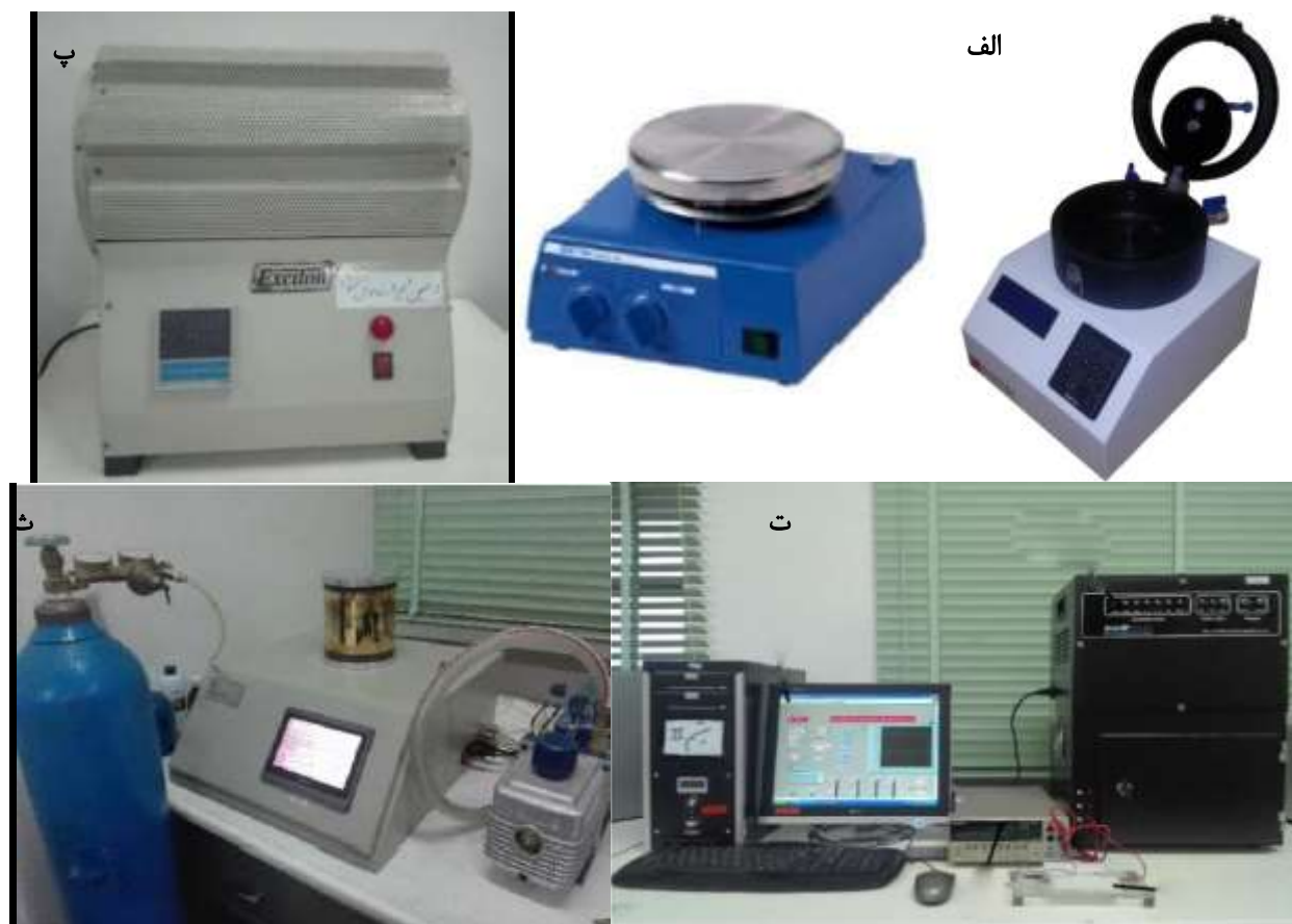
شکل ۲ وسایل مورد استفاده الف- دستگاه لایه‌نشانی چرخشی ب- کوره افقی پ- گرم کننده ت- دستگاه شبیه‌ساز نور خورشید و مشخصه‌یابی جریان-ولتاژ ث- دستگاه کند و پاش.
