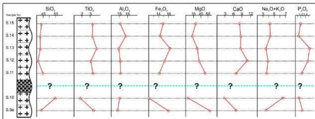
شکل ۶ نمودار تغییر مقادیر اکسیدهای عناصر اصلی در توالی نمونه‌های برداشت شده (بدون مقیاس). علامت ؟ مربوط به نمونه آب‌آواری (شکل ۲-ت) است.
