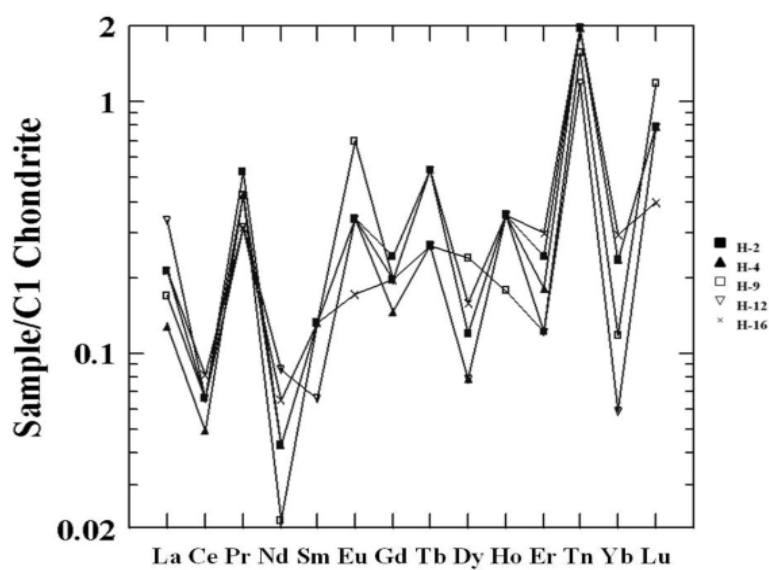
شکل ۱۴ مقادیر پهنجار شده عناصر کمیاب شاخص‌های کرومیت منطقه نیریز نسبت به کندریت C 1 [۳۰].
