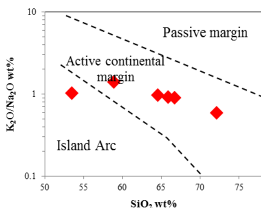
شکل ۳ الف: نمودار \log \text{Fe}_2\text{O}_3/\text{K}_2\text{O} نسبت به \log \text{SiO}_2/\text{Al}_2\text{O}_3 [۱۱]، که نشان‌دهنده ترکیب شیل و ماسه سنگ تیره شیت‌های گل‌گهر است. ب: نمودار تجزیه‌ای \text{K}_2\text{O}/\text{Na}_2\text{O} نسبت به \text{SiO}_2 [۱۲]، جهت شناسایی جایگاه زمین‌ساختی شیت‌های مورد بررسی.
