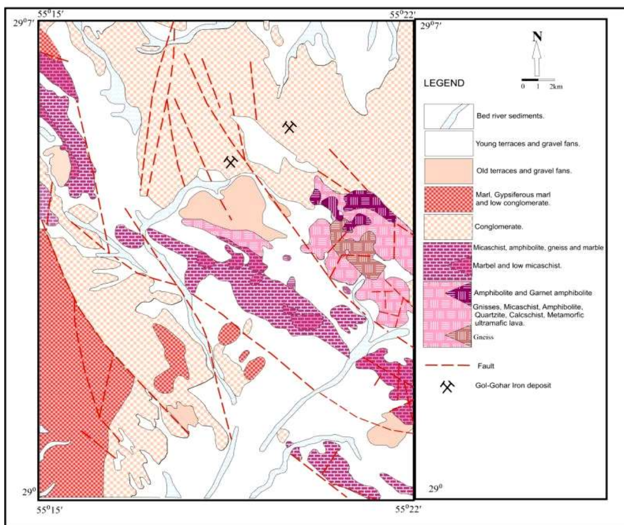
شکل ۱ نقشه زمین‌شناسی ناحیه‌ای ساده شده از منطقه گل‌گهر (برگرفته از نقشه ۱/۱۰۰۰۰۰ گل‌گهر [۸] با تغییرات).
