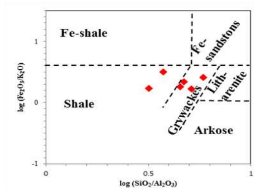
شکل ۳ الف: نمودار \log \text{Fe}_2\text{O}_3/\text{K}_2\text{O} نسبت به \log \text{SiO}_2/\text{Al}_2\text{O}_3 [۱۱]، که نشان‌دهنده ترکیب شیل و ماسه سنگ تیره شیت‌های گل‌گهر است. ب: نمودار تجزیه‌ای \text{K}_2\text{O}/\text{Na}_2\text{O} نسبت به \text{SiO}_2 [۱۲]، جهت شناسایی جایگاه زمین‌ساختی شیت‌های مورد بررسی.
