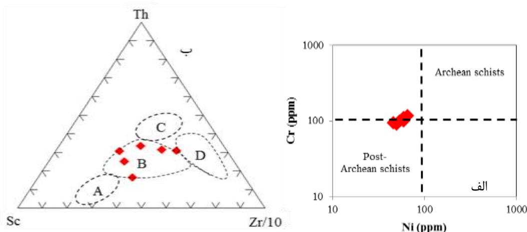
شکل ۴ الف: نمودار دوتایی Ni-Cr برای شیت‌های مورد بررسی. میدان‌های مشخص شده برای شیت‌های آرکئن و پس از آرکئن برگرفته از مرجع [۱۳] است. ب: نمودار سه تایی Sc-Th-Zr/10 برای شیت‌های مورد بررسی. گستره‌های مشخص شده عبارتند از: A: جزایر کمانی اقیانوسی، B: جزایر کمانی قاره‌ای، C: کرانه فعال قاره‌ای و D: کرانه غیر فعال [۱۶]. پ: ترکیب نمونه‌های گل‌گهر بر نمودار SiO 2 نسبت به K 2 O [۱۷].
