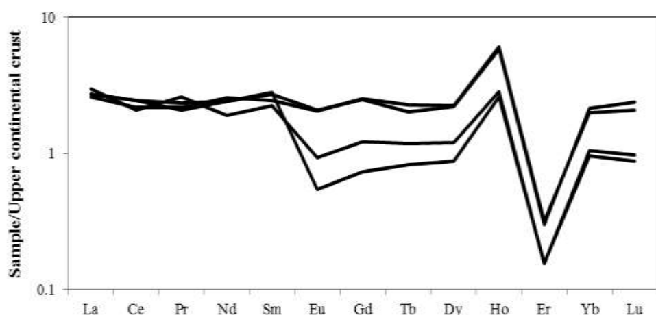
شکل ۸ الگوی پراکندگی عناصر خاکی نادر بهنجار شده نسبت به پوسته قاره‌ای بالایی [۳۰] در گنیس‌های منطقه گل‌گهر.
