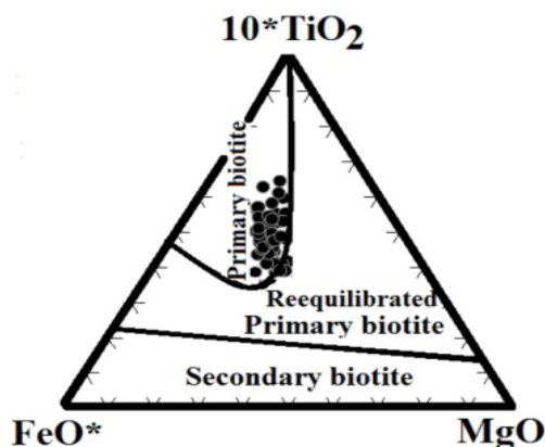
شکل ۶ نمودار سه تایی \text{MgO} ، 10\text{TiO}_2 ، \text{FeO}^* که بیوتیت‌های اولیه و بیوتیت‌های که دستخوش تعادل مجدد در محیط شده‌اند را از بیوتیت‌های ثانوی متمایز می‌سازد.
