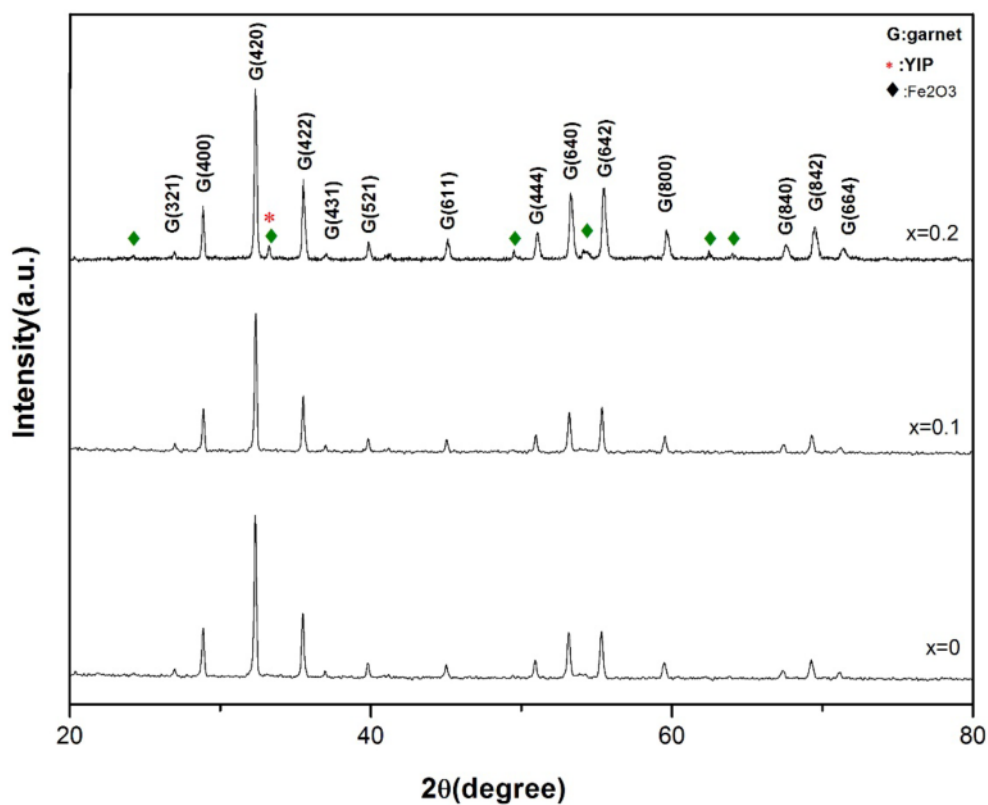
شکل ۱ الگوهای پراش پرتو ایکس نانوذرات گارنت \text{Bi}_{0.5}\text{Y}_{2.5-x}\text{Fe}_{5+x}\text{O}_{12} با مقدار جانشانی گوناگون ( x = 0, 0.1, 0.2 ).
