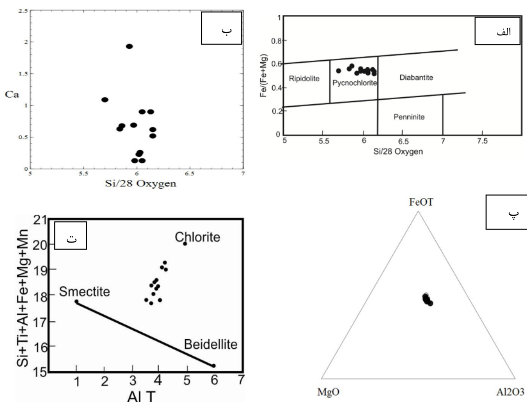
شکل ۴ نمونه‌های مورد بررسی بر الف) نمودار رده‌بندی کلریت‌ها [۱۳] و ب) نمودار Ca-Si، پ- نمونه کلریت‌های مورد بررسی بر نمودار MgO- FeO_T - Al_2O_3 (ت) گستره ترکیبی کلریت‌های مورد بررسی [۳۰]، این کلریت‌ها دارای لایه‌هایی از کانی‌های اسمکتیت هستند.
