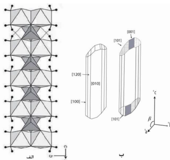
شکل ۳ الف) ساختار سه‌بعدی بلور اریثرایت، که هرم‌های خاکستری تیره چاروجهی‌های آرسنیک، هشت‌وجهی‌های خاکستری روشن کبالت و آهن، دایره‌های سیاه، اتم‌های هیدروژن و خطوط تیره پیوند اکسیژن به هیدروژن را نشان می‌دهند. ب) سیستم و محورهای بلورشناسی کانی-اریثرایت (برگرفته از [۱۰، ۱۳]).
