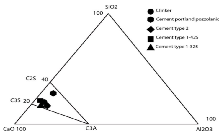
شکل ۴ موقعیت ترسیمی سیمان نوع ۱-۴۲۵، سیمان نوع ۲، سیمان پرتلند پوزولانی، سیمان نوع ۱-۳۲۵ و کلینکر در سیستم فازی C-S-A [۱۱]. C_3S نشان دهنده فاز آلیت، C_2S نشان دهنده فاز بلیت و C_3A نشان دهنده فاز تری‌کلسیم آلومینات هستند.
