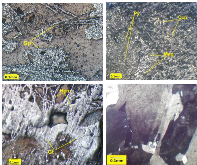
شکل ۸ الف تصویر میکروسکوپی از مگنتیت (Mag) به همراه پیریت (Py) و کالکوپیریت (Ccp) درون منطقه‌ی اسکارنی نور PPL، ب) تصویر میکروسکوپی از اسپیکولاریت نور PPL، پ) تصویر میکروسکوپی از باریت نور XPL، ت) تصویر میکروسکوپی گوتیت (Gt) با بافت کلوفرم و هماتیت (Hem) در نور PPL [۲۰].
