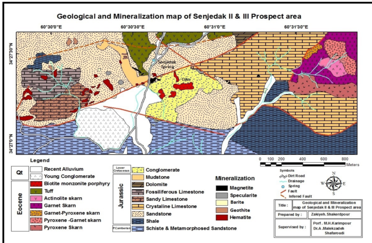
شکل ۳ نقشه‌ی زمین‌شناسی و کانی‌سازی مناطق پی‌جویی سنجدک II و III [۱۲].
