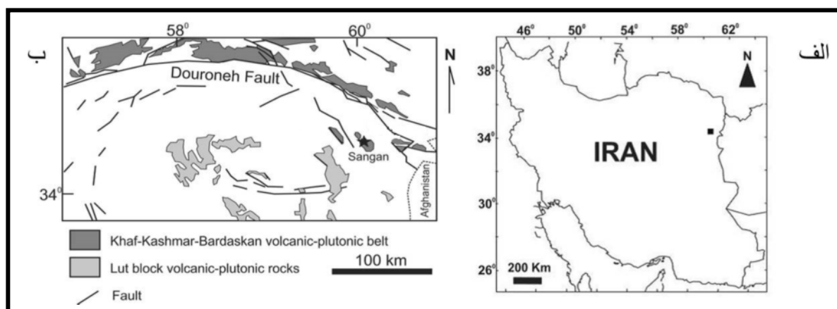
شکل ۱ الف) موقعیت جغرافیایی معدن سنگان در شمال شرقی ایران، ب) موقعیت معدن سنگان در کمربند ماگایی خواف-کاشمر- بردسکن.
