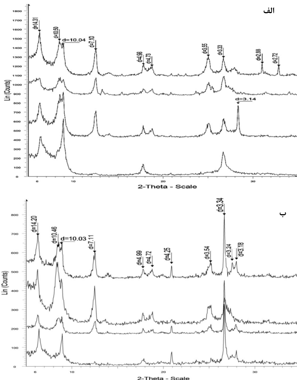
شکل ۲ الگوهای XRD رس‌های آرایش یافته مربوط به الف: افق A و ب: افق C۱ نیمرخ زمین بایر (اعداد ارائه شده بر قله‌ها فاصله بین صفحه‌ای بر حسب آنگستروم و طیف‌ها از بالا به پایین به ترتیب مربوط به تیمار منیزیم، منیزیم و گلیسرول، پتاسیم و تیمار پتاسیم و گرمای ۵۵۰ درجه سانتی‌گراد هستند).
