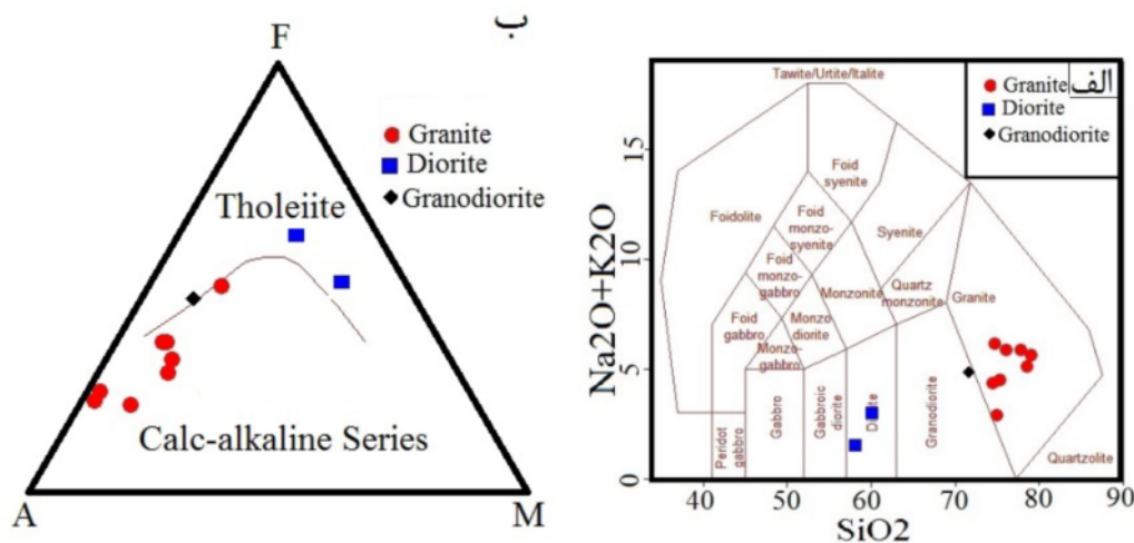
شکل ۵. موقعیت نمونه‌های مورد بررسی در \text{SiO}_2 (الف) برابر [\text{Na}_2\text{O} + \text{K}_2\text{O}] (ب)، AFM [۱۱]
