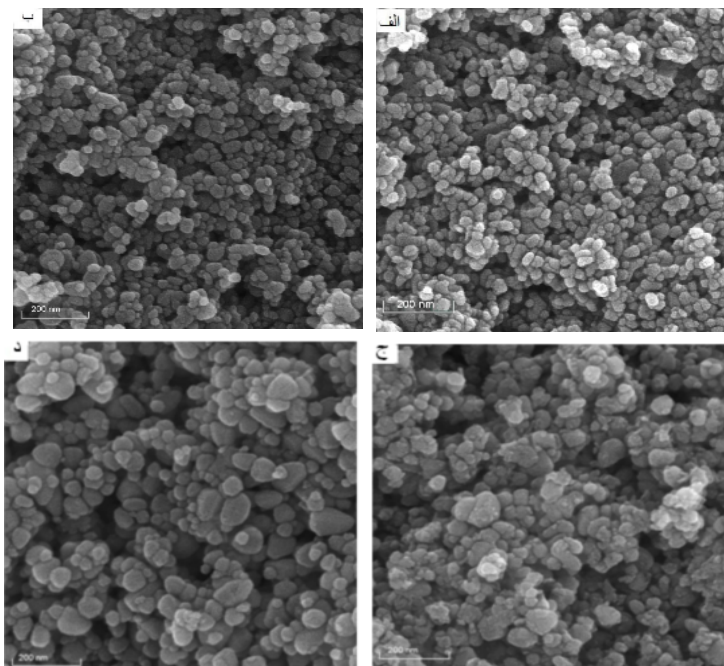
شکل ۲ تصاویر FESEM نمونه‌های Zn_{1-x}Ni_xO (الف) x=0 (ب) x=0.1 (ج) x=0.2 (د) x=0.3 .
