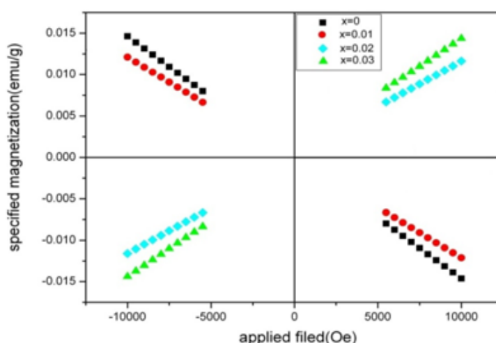
شکل ۸. نتایج VSM نمونه‌های \text{Zn}_{1-x}\text{Ni}_x\text{O} در میدان‌های قوی.
