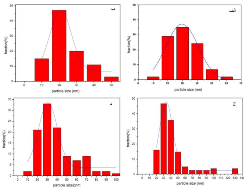
شکل ۳ توزیع اندازه‌ی ذرات نمونه‌های Zn_{1-x}Ni_xO (الف) x=0 (ب) x=0.1 (ج) x=0.2 (د) x=0.3 .
