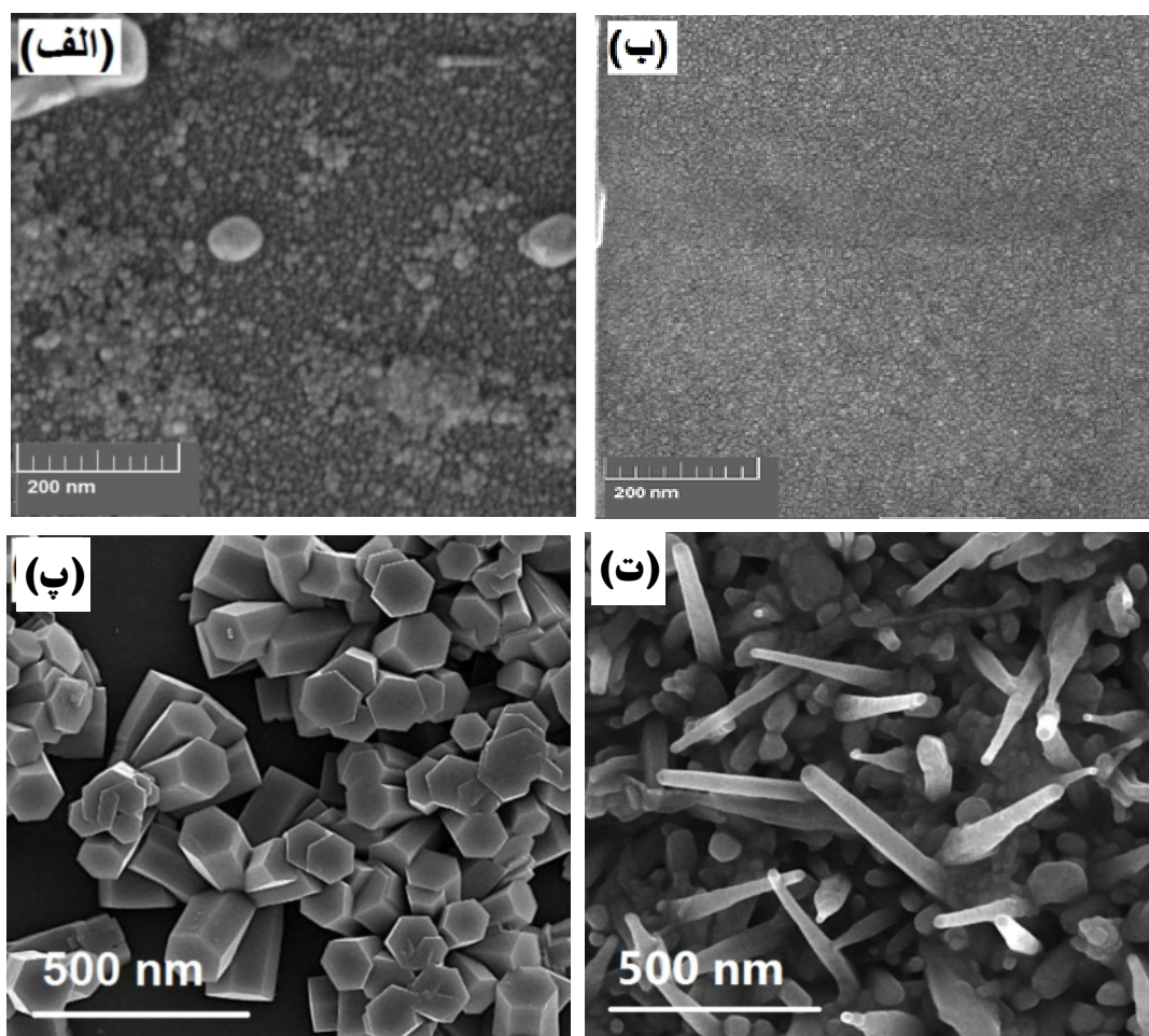
شکل ۳ تصاویر FESEM لایه‌ی بذر نمونه‌ی (الف) نمونه‌ی (ب) و نانومیله‌های اکسید روی با غلظت محلول ۲۵ mM رشد یافته بر لایه‌ی بذر نمونه‌ی (الف، پ) نمونه‌ی (ت). (ب) و نانومیله‌های اکسید روی با غلظت محلول ۲۵ mM رشد یافته بر لایه‌ی بذر
