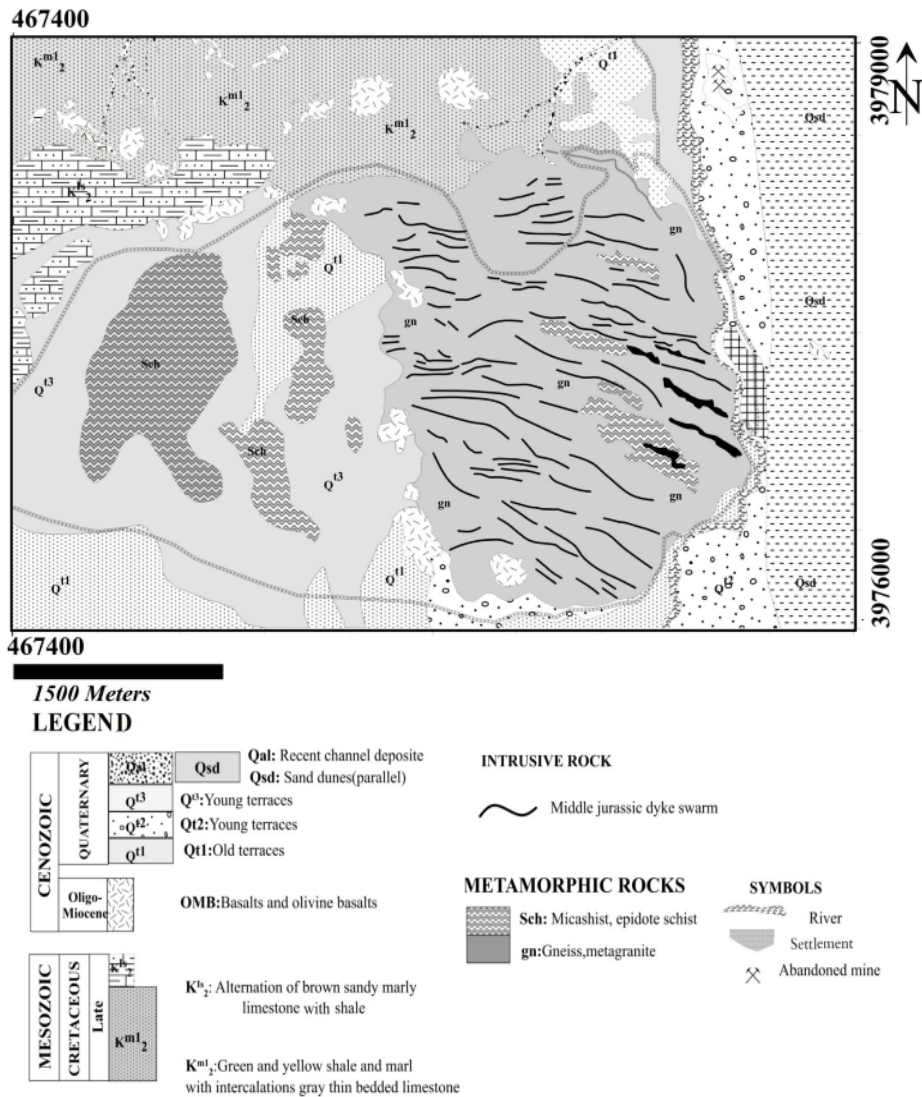
شکل ۱ نقشه زمین شناسی دایک‌های دیابازی منطقه رضاآباد (جنوب غربی بیارجمند).
