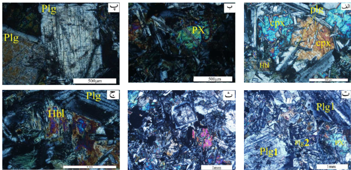
شکل ۴ الف) نمایش بافت افیتی و نیمه افیتی در دایک‌های دیابازی (ب) تصویری از بلور کلینوپیروکسن با ماکل اوزیتی (XPL)، (پ) ماکل پلی- سنتتیک در پلاژیوکلازها (XPL)، (ت) تصویری از وجود دو نسل پلاژیوکلاز در نمونه‌های دیابازی (XPL). (ث) منطقه‌بندی در درشت بلور پلاژیوکلازهای نسل اول (XPL)، (ج) تصویری از کانی هورنبلند در دایک‌های دیابازی که در حال تبدیل شدن به کلریت است (XPL).
