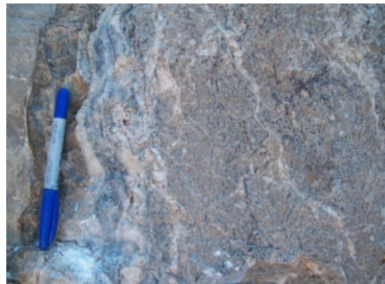
شکل ۱۵: بافت برشی خرد شده شامل قطعات خرد شده سنگ میزبان و سیمان ماده معدنی.
