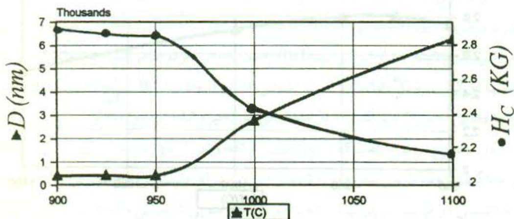
شکل ۲ وابستگی اندازه دانه‌بندی، D و میدان وادارنده مغناطیسی، H_c به دمای تفجوشی نمونه‌ها.
