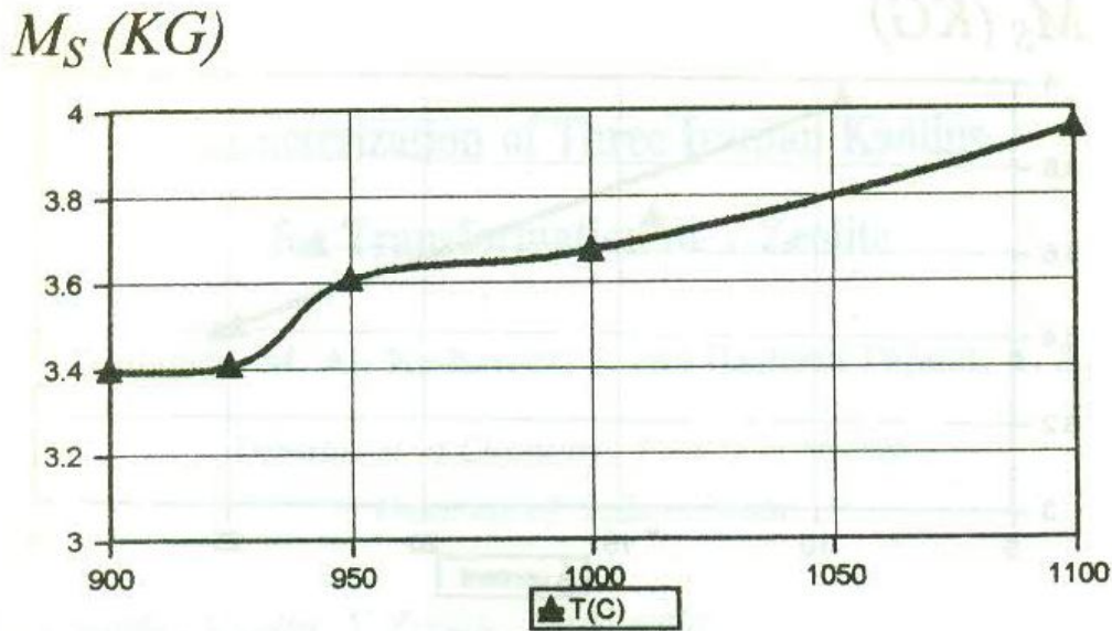
شکل ۵ وابستگی مغناطش اشباع، M_s به دمای تفجوشی نمونه.
