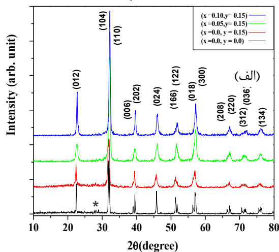
شکل ۱ الگوی پراش پرتو ایکس نانوذرات BB_yL_xFO در دمای اتاق. الف) طیف در گستره‌ی زوایای 20 \leq \theta \leq 80 ، ب) بزرگنمایی طیف و جابجایی قله به سمت زوایای بزرگتر در 20 \leq \theta \leq 33 .
