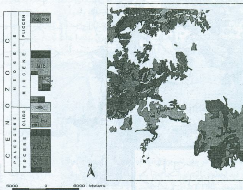
شکل ۲ نقشه واحدهای سنگی منطقه میانه که با تصاویر ماهواره‌ای تصحیح شده و از ته‌نشتهای دوره‌های بعدی چشم پوشی شده است (مختصات عینا مشابه شکل ۱ است).
