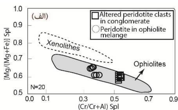
شکل ۴ (الف) نمودار Mg/(Mg+Fe) نسبت به Cr/(Cr+Al) در اسپینل [۱۶، ۱۷]، (ب) نمودار درصد وزنی Al_2O_3 نسبت به Cr_2O_3 اسپینل [۱۸]. ترکیب اسپینل در پریدوتیت‌های مجموعه‌ی افیولیتی پیرانشهر برای مقایسه در نمودار تصویر شده است. ترکیب اسپینل در قطعات پریدوتیت دگرسان شده درون کنگلومرا و پریدوتیت‌های ملائز افیولیتی پیرانشهر در گستره‌ی آرایه‌ی گوشته‌ای قرار می‌گیرند.
