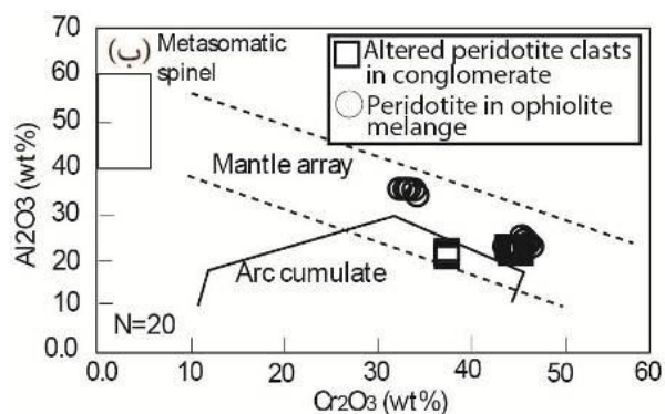
شکل ۴ (الف) نمودار Mg/(Mg+Fe) نسبت به Cr/(Cr+Al) در اسپینل [۱۶، ۱۷]، (ب) نمودار درصد وزنی Al_2O_3 نسبت به Cr_2O_3 اسپینل [۱۸]. ترکیب اسپینل در پریدوتیت‌های مجموعه‌ی افیولیتی پیرانشهر برای مقایسه در نمودار تصویر شده است. ترکیب اسپینل در قطعات پریدوتیت دگرسان شده درون کنگلومرا و پریدوتیت‌های ملائز افیولیتی پیرانشهر در گستره‌ی آرایه‌ی گوشته‌ای قرار می‌گیرند.
