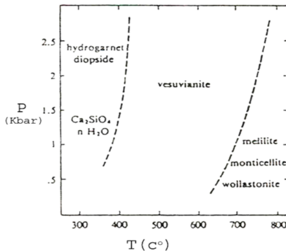
نمودار ۲ منحنی P-T تشکیل وزوویانیت در محیطی با آب خالص و عاری از آلکالی برای ترکیب ژل \text{Ca}_{20}\text{Al}_8\text{Mg}_4\text{Si}_8(\text{OH})_{6.n}\text{H}_2\text{O} (اقتباس از [۱۴]).
