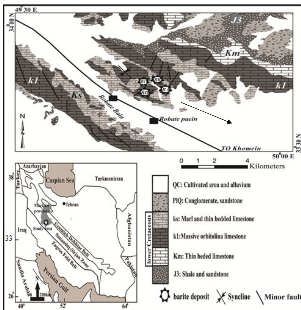
شکل ۲ موقعیت واحدهای ساختاری اصلی ایران و جایگاه منطقه‌ی مورد بررسی اقباس [۴] و نقشه‌ی زمین‌شناسی ساده‌شده‌ی گستره‌ی کانسار باریت رباط پائین [۵].
