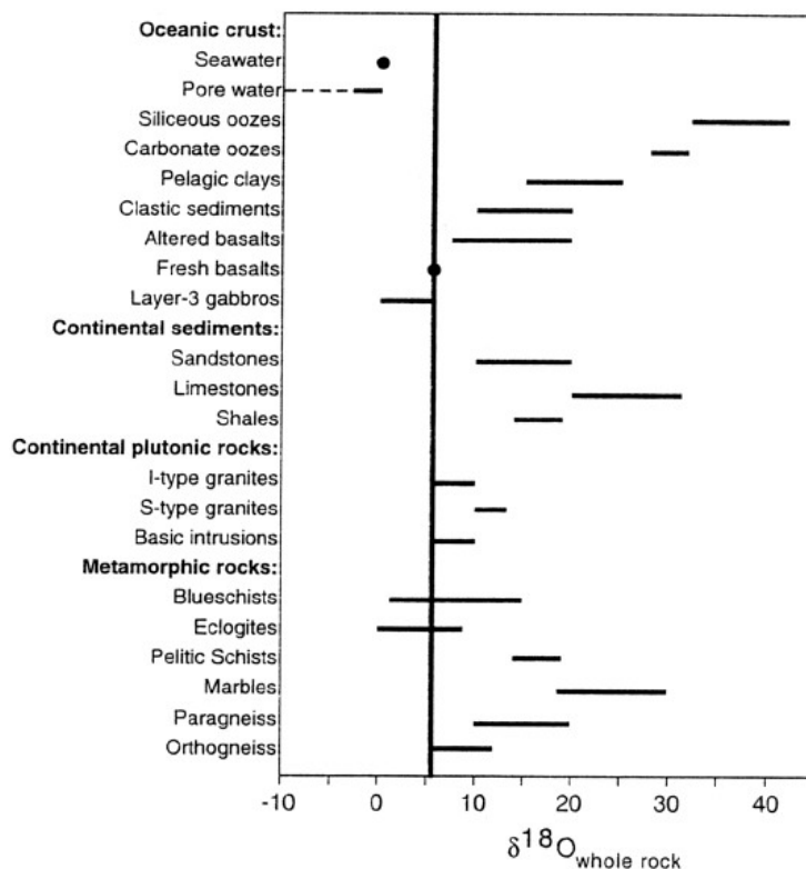
شکل ۷ نمودار مقادیر ایزوتوپی اکسیژن در سنگهای مختلف. در این نمودار مقادیر ایزوتوپی رگه‌های مورد مطالعه (۱۳ تا ۱۷ ‰ \delta^{18}\text{O} در مقایسه با استاندارد SMOW) تقریباً مشابه مقادیر مربوط به شیستهای پلیتی است. اقتباس از [۲۵].
