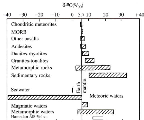
شکل ۶ مقایسه مقادیر ایزوتوپهای اکسیژن در سنگها، آبهای طبیعی و رگه‌های آلومینوسیلیکات‌دار منطقه همدان در مقایسه با استاندارد SMOW. اقتباس شده از [۲۴] به نقل از [۲ و ۳].
